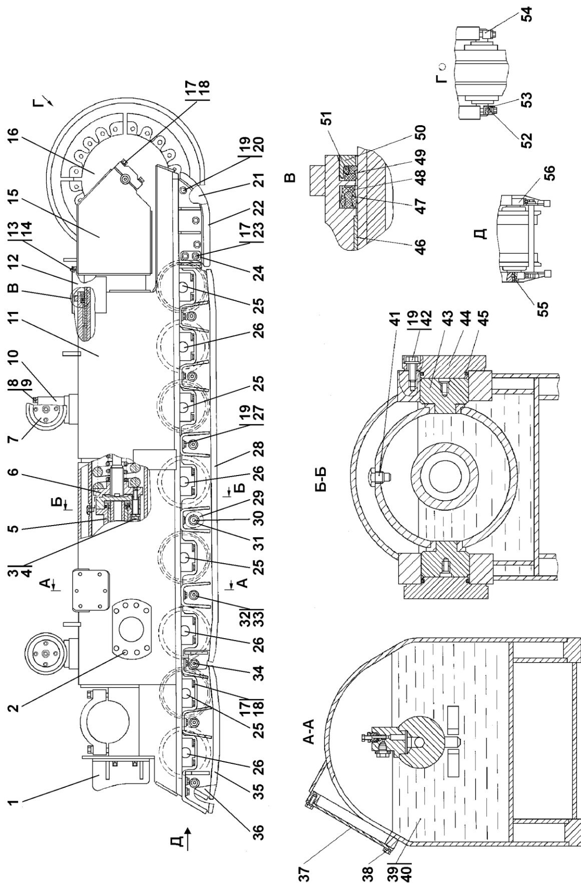
Рисунок 8.8 Тележка Figure 8.8 Bogie
