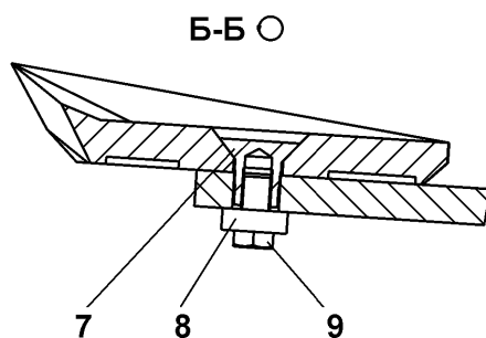
Рисунок 8.18 Отвал Figure 8.18 Blade
