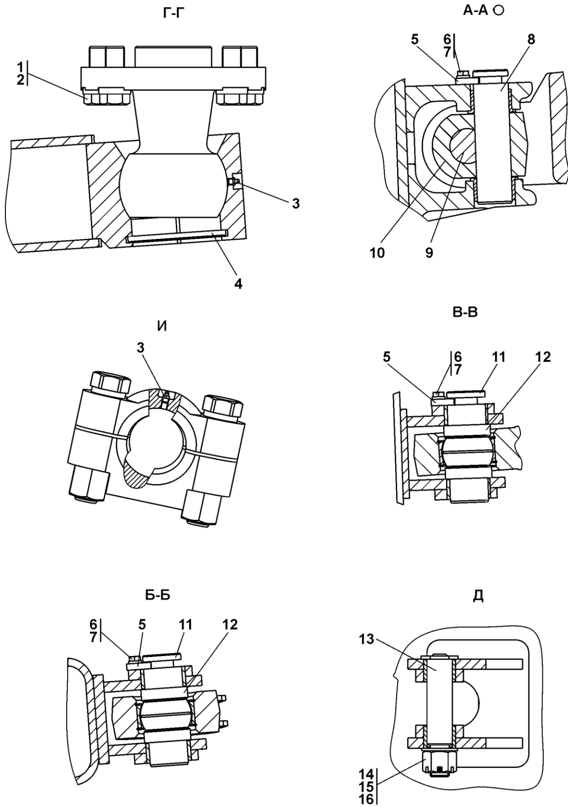
Рисунок 8.17 Оборудование бульдозерное полусферическое Figure 8.17 Hemispherical dozer equipment
