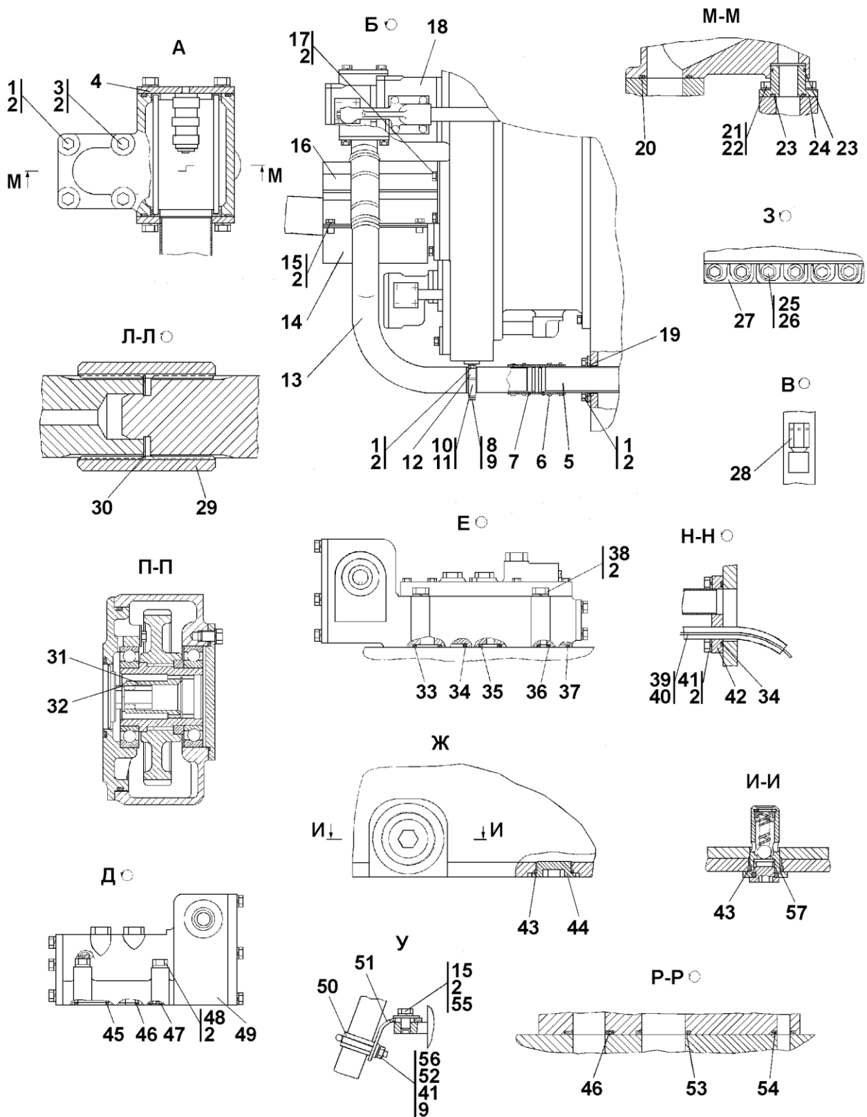
Рисунок 8.4 Установка трансмиссии Figure 8.4 Transmission mounting
