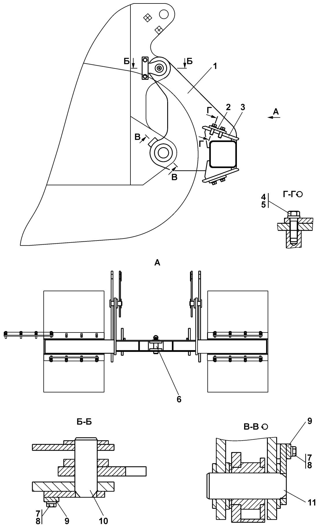
Рисунок 8.21 Отбойник с прицепным устройством Figure 8.21 Impingement plate with the hitch
