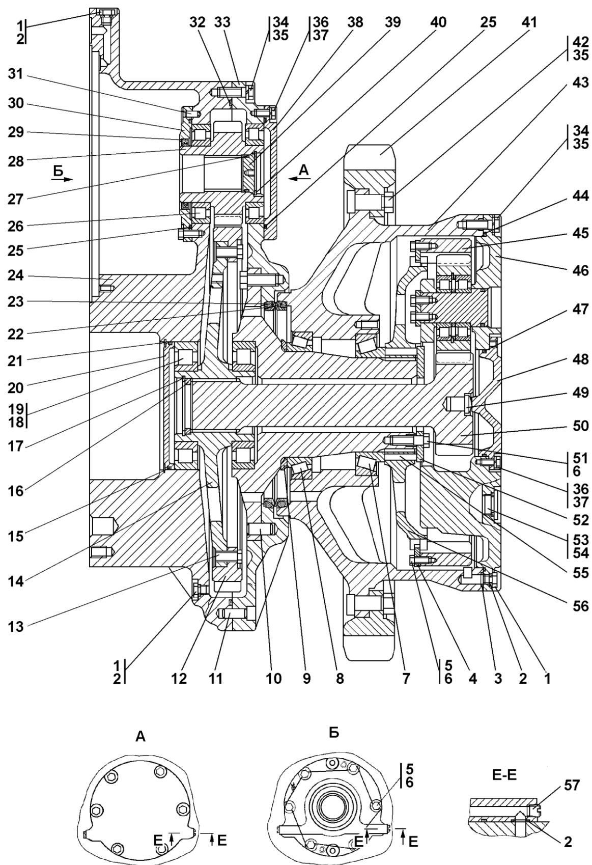
Рисунок 8.6 Передача бортовая Figure 8.6 Final drive
