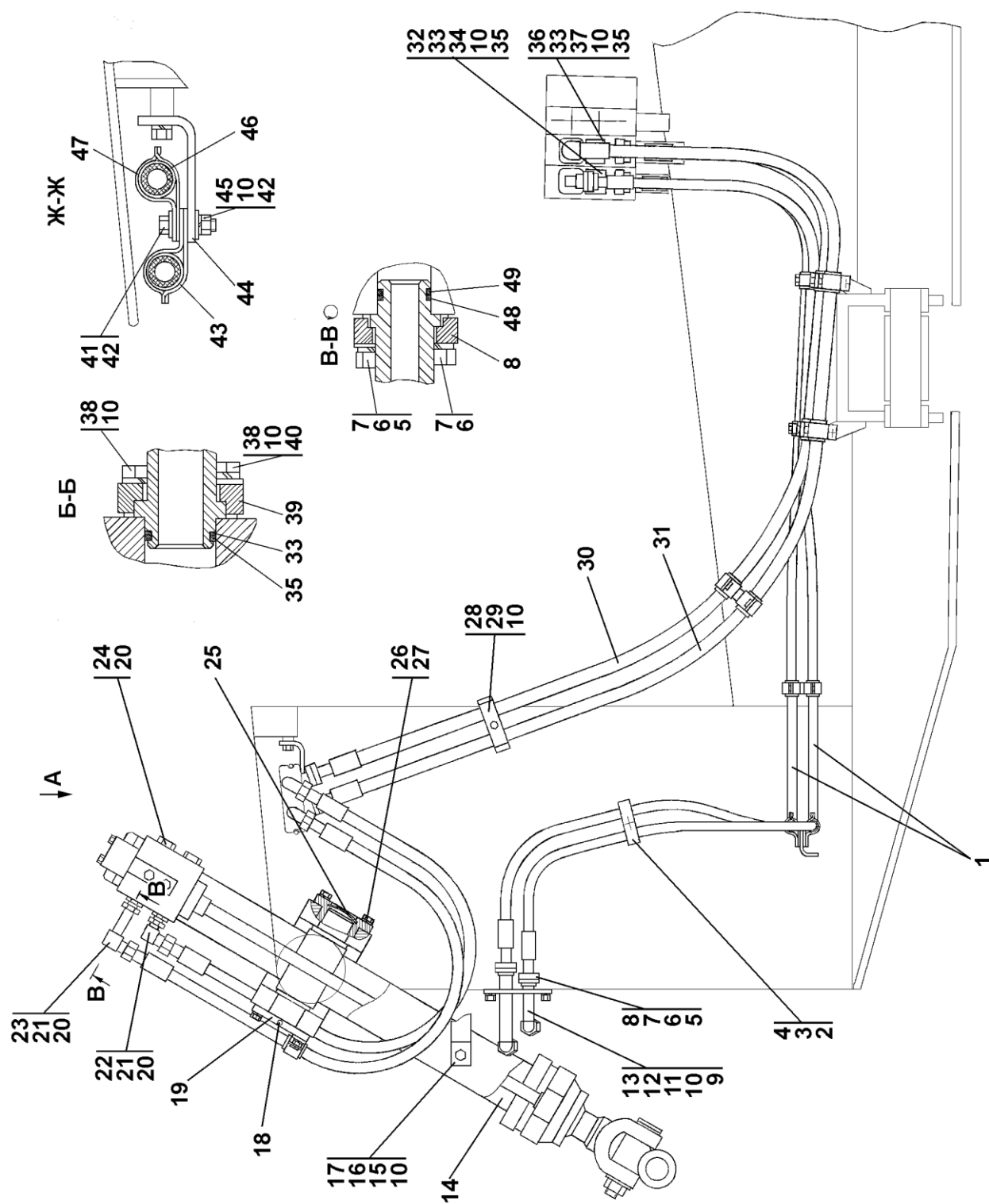
Рисунок 8.11 Установка гидроцилиндров Figure 8.11 Hydraulic cylinders mounting
