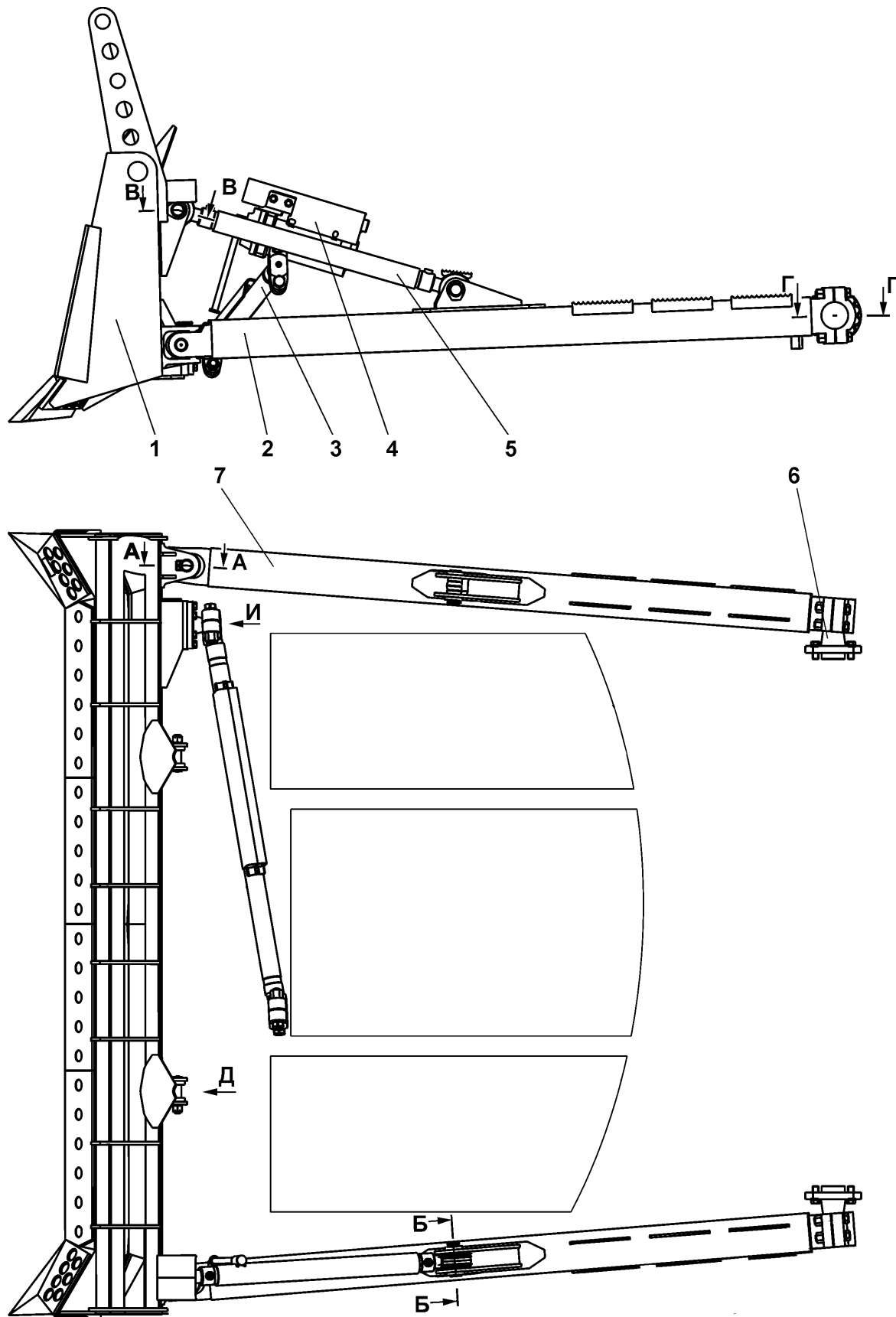
Рисунок 8.16 Оборудование бульдозерное полусферическое Figure 8.16 Hemispherical dozer equipment
