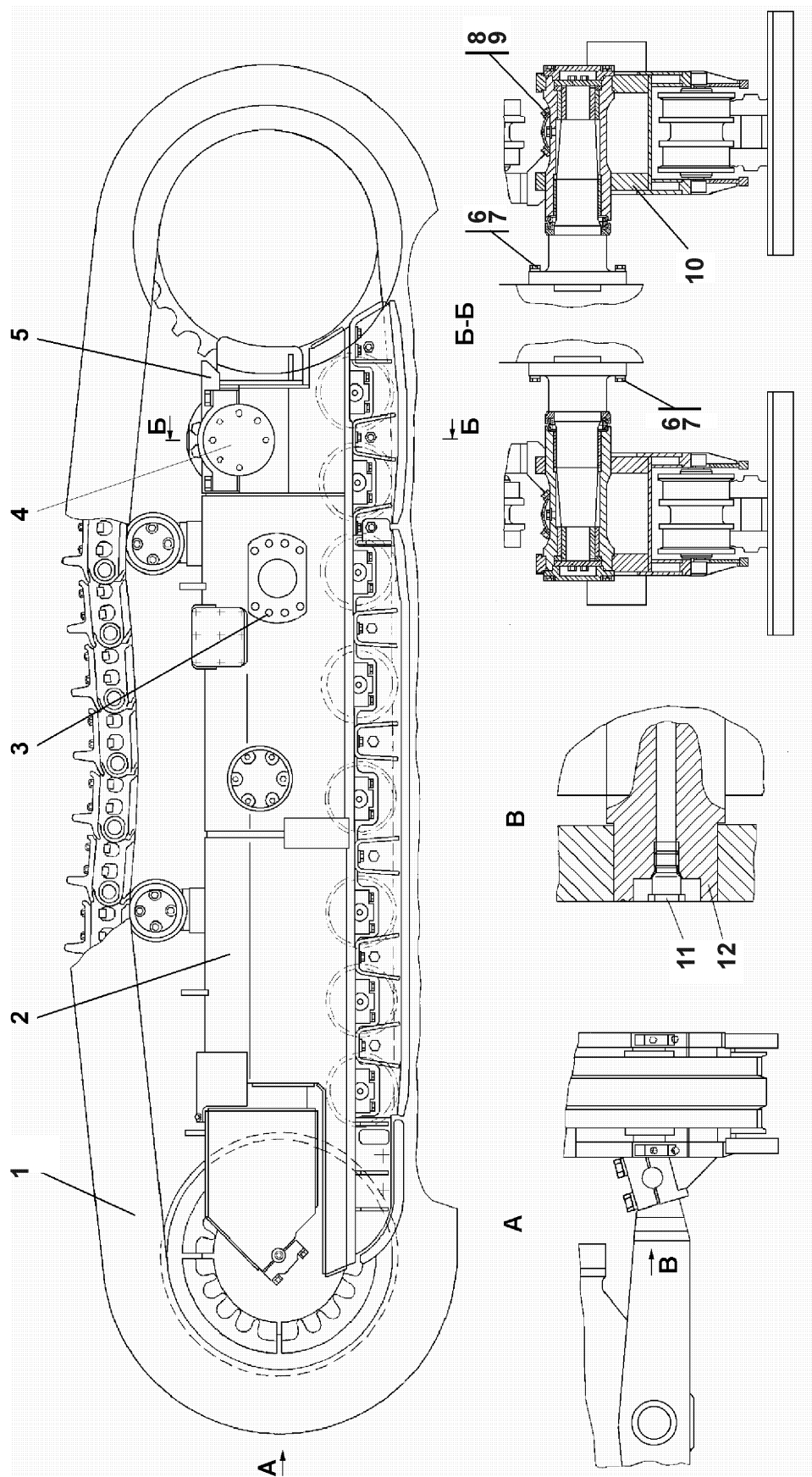
Рисунок 8.7 Система ходовая Figure 8.7 Running gear
