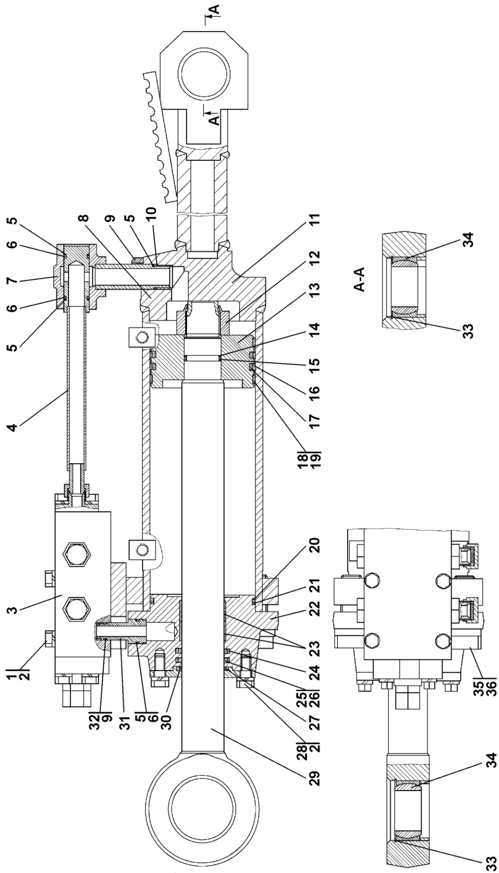
Рисунок 8.20 Гидрораскос Ø160 Figure 8.20 Hydraulic brace Ø160
