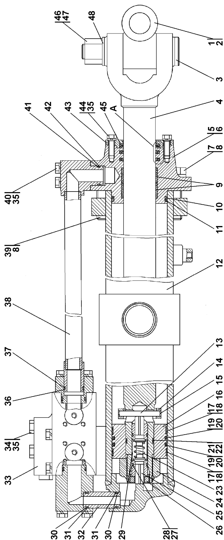
Рисунок 8.13 Гидроцилиндр Ø110 Figure 8.13 Hydraulic cylinder Ø110
