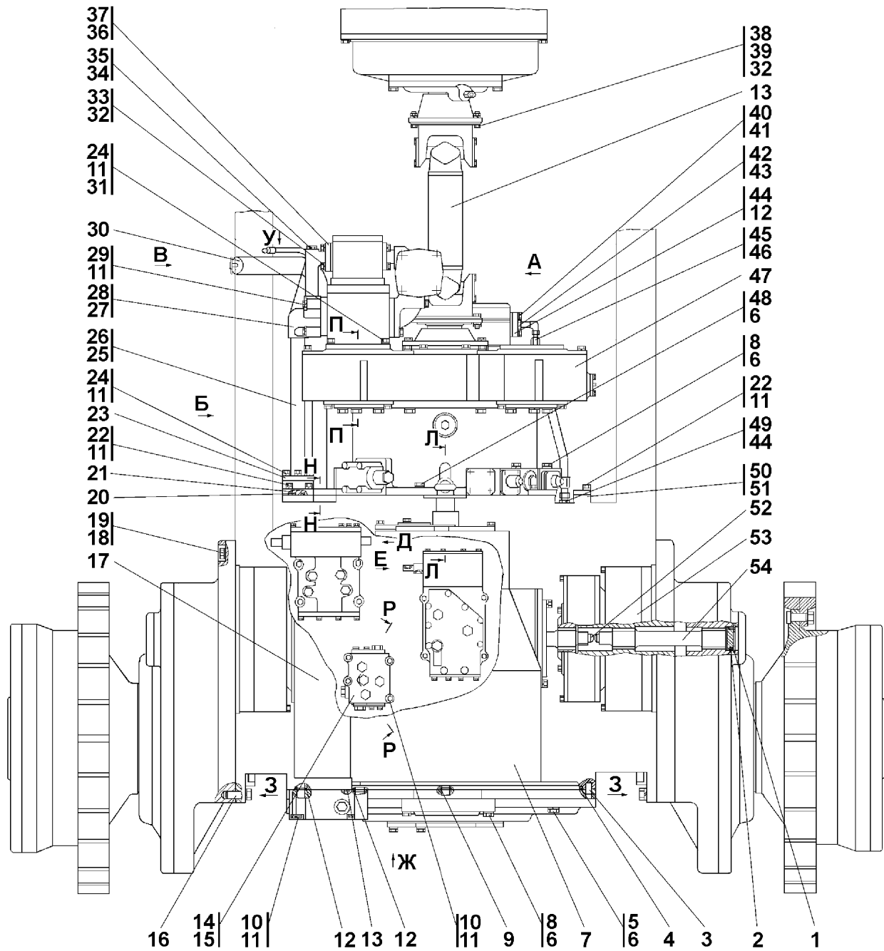
Рисунок 8.3 Установка трансмиссии Figure 8.3 Transmission mounting
