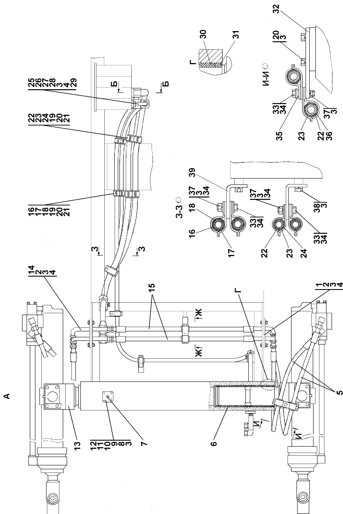
Рисунок 8.12 Установка гидроцилиндров Figure 8.12 Hydraulic cylinders mounting
