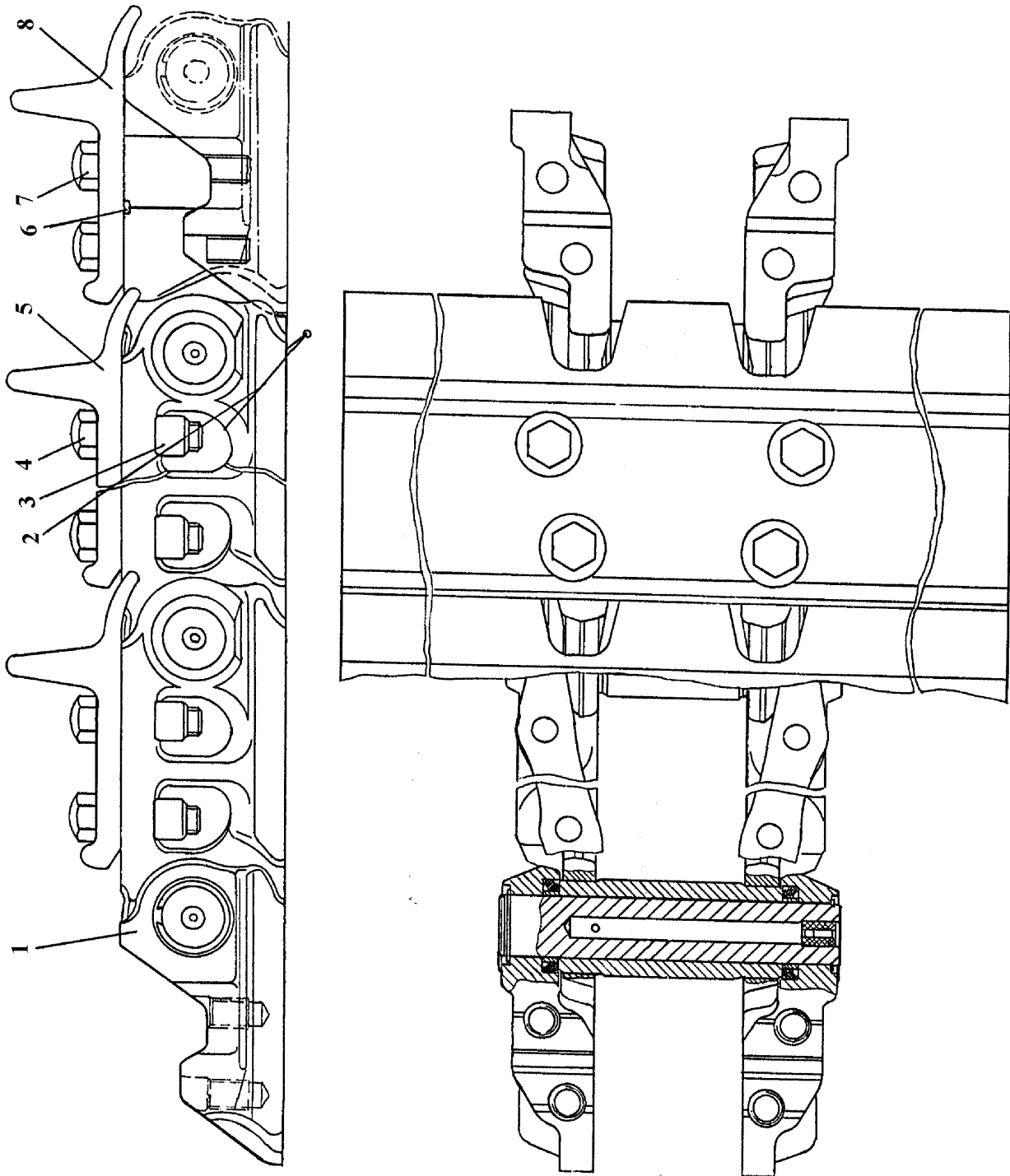
Рисунок 8.10 Гусеница Figure 8.10 Track
