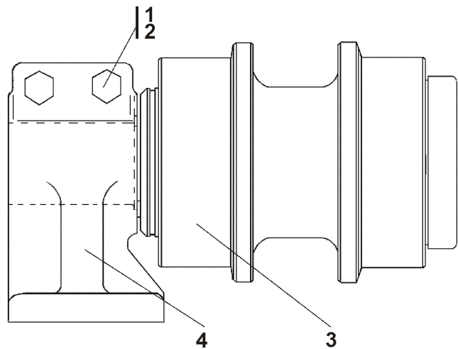
Рисунок 3.9 Каток поддерживающий Figure 3.9 Support roller
