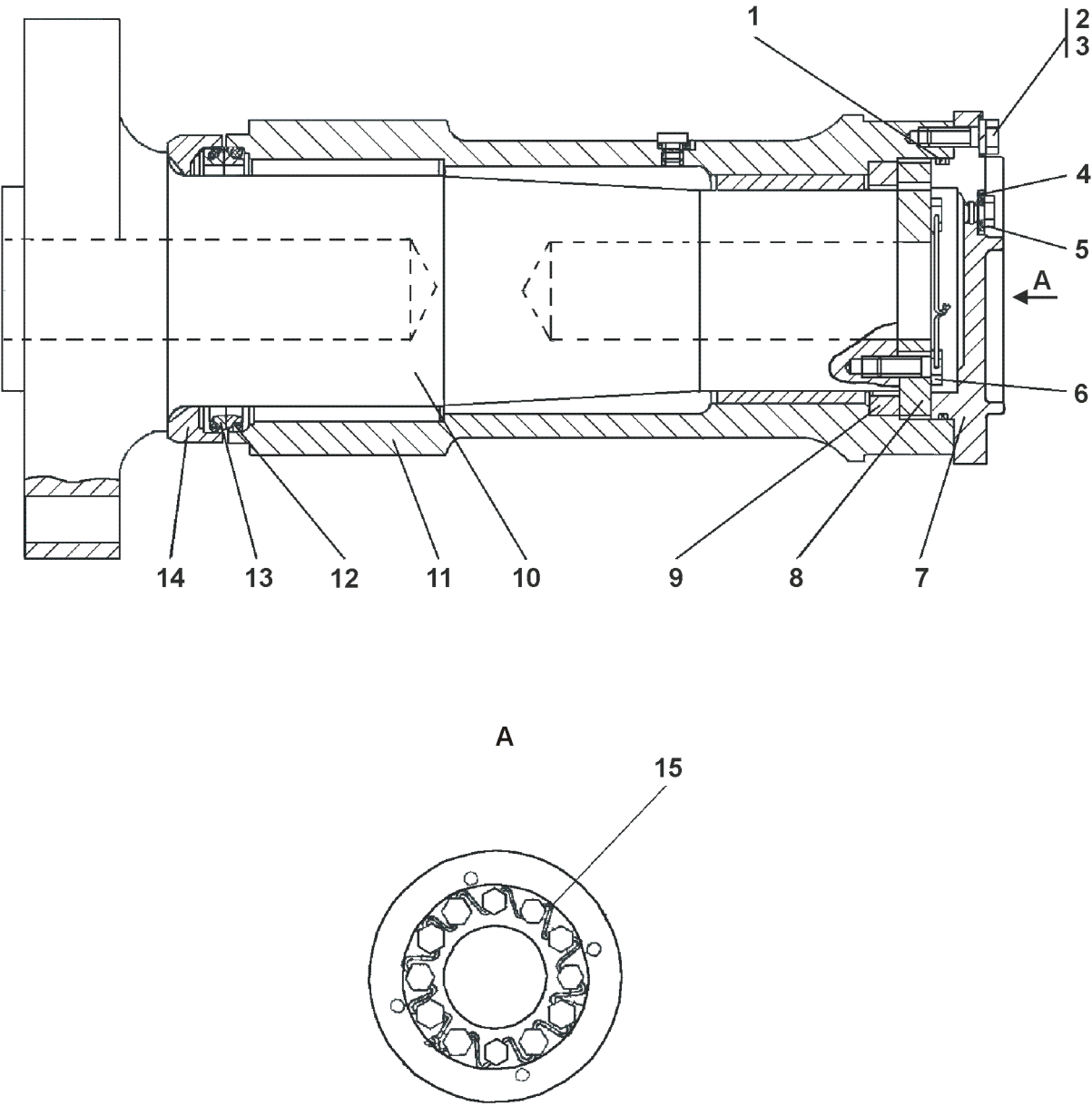
Рисунок 3.7 Шарнир Figure 3.7 Hinge
