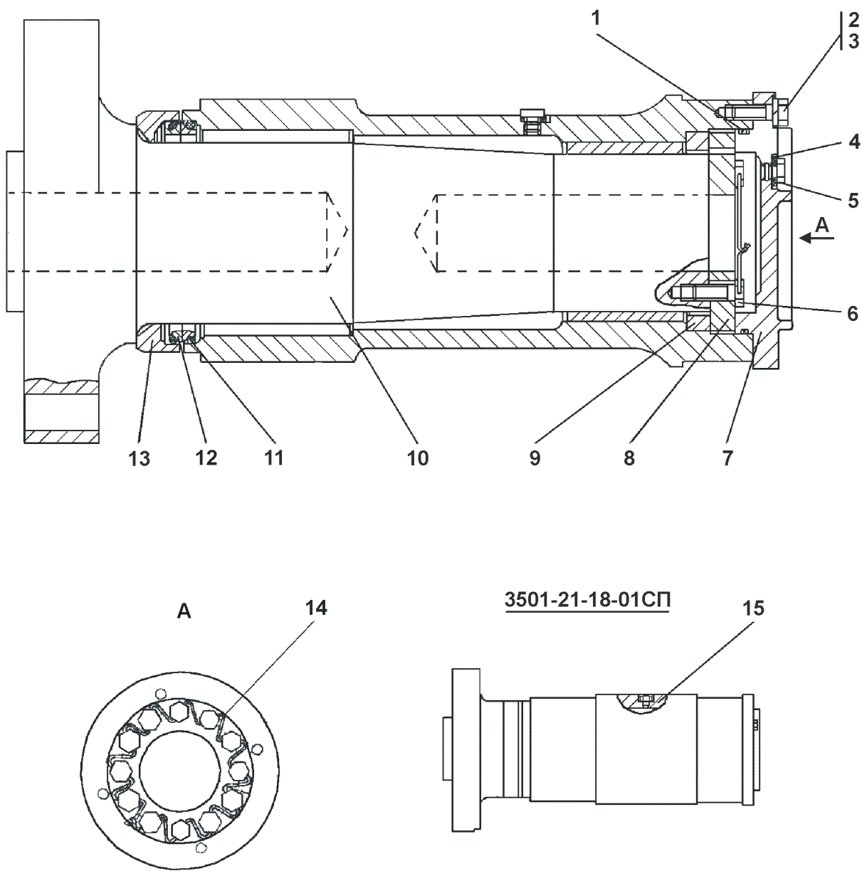
Рисунок 3.8 Шарнир Figure 3.8 Hinge
