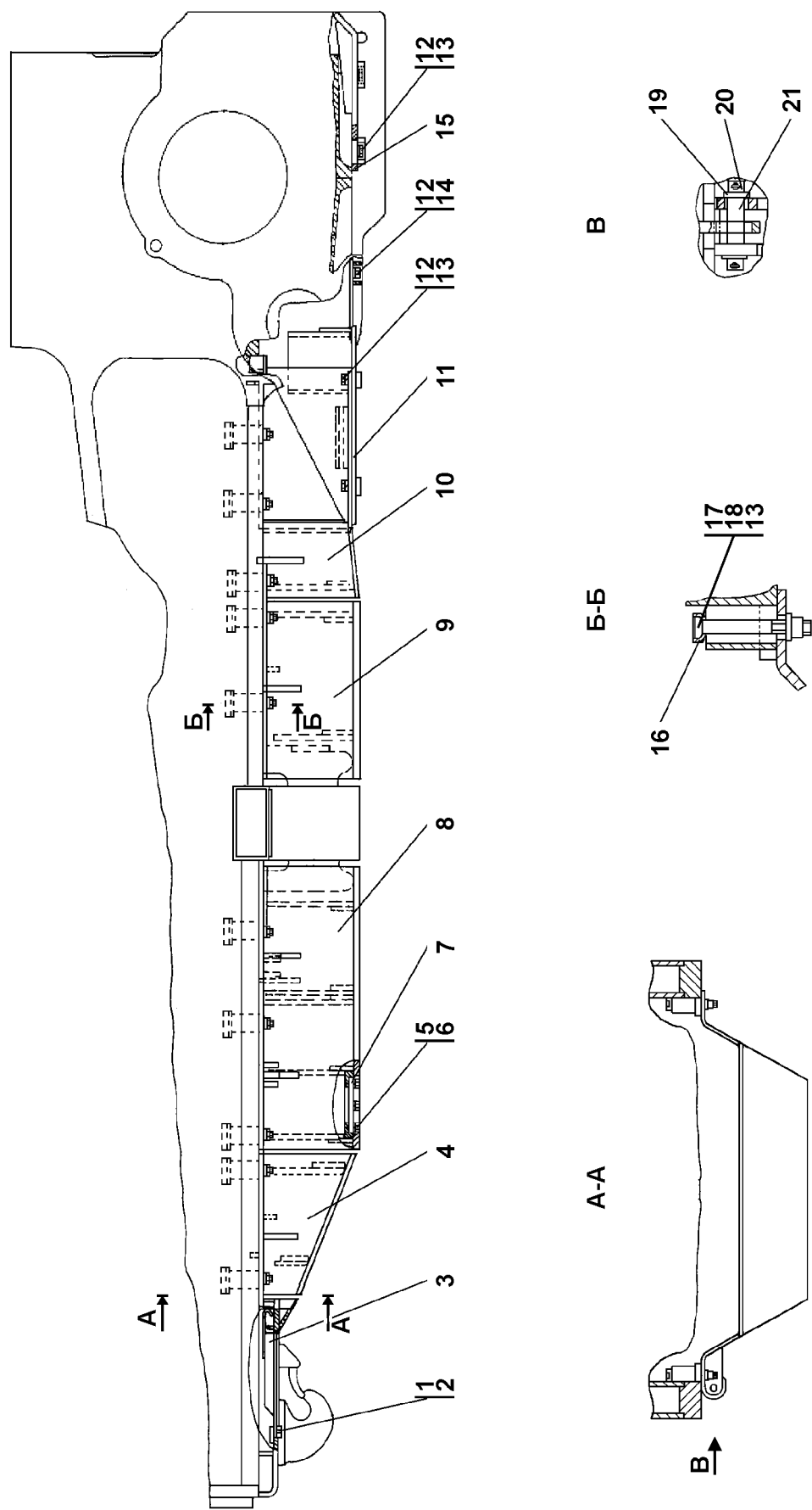
Рисунок 3.16 Установка кожухов Figure 3.16 Jackets mounting
