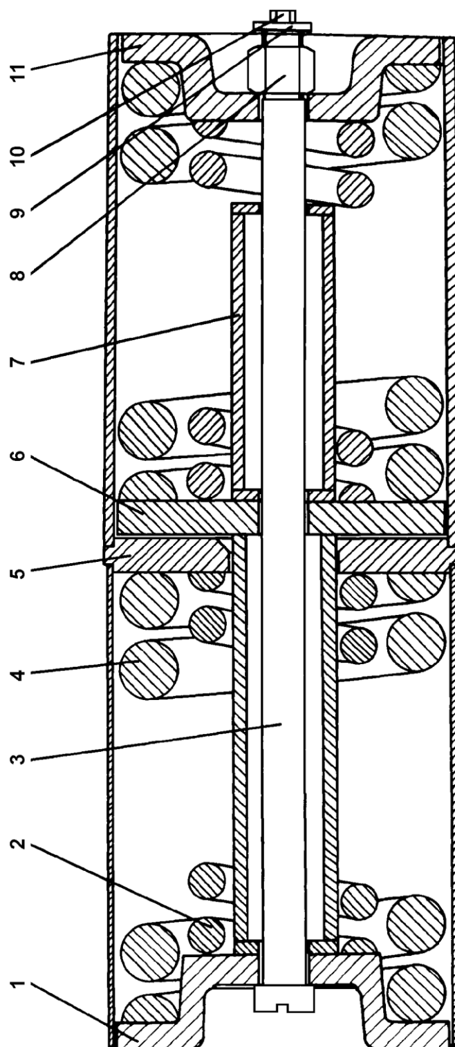
Рисунок 3.12 Механизм сдвигания Figure 3.12 Recoil mechanism
