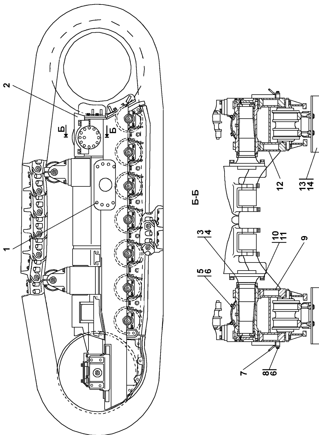
Рисунок 3.3 Система ходовая Figure 3.3 Running gear
