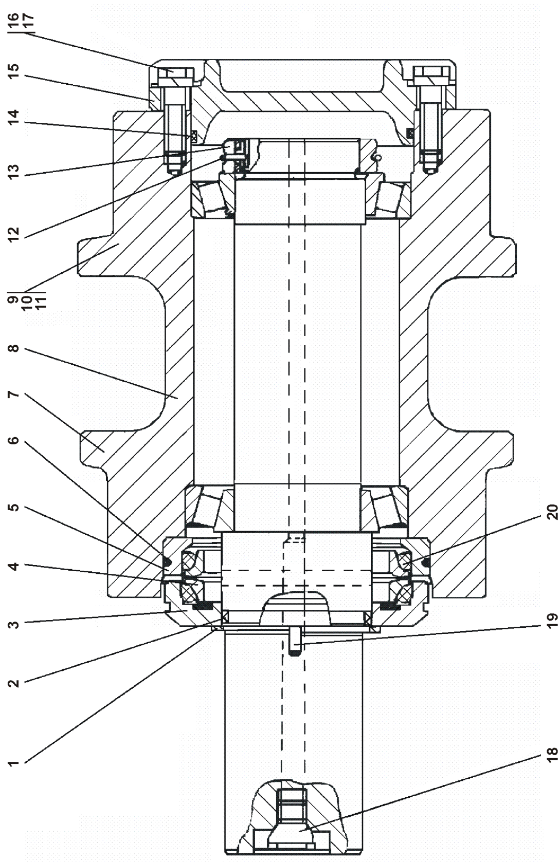
Рисунок 3.10 Каток поддерживающий Figure 3.10 Support roller
