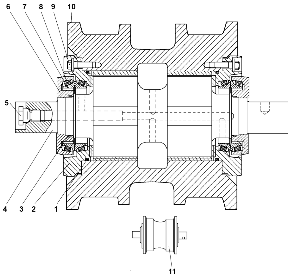
Рисунок 3.7 Каток опорный Figure 3.7 Support roller
