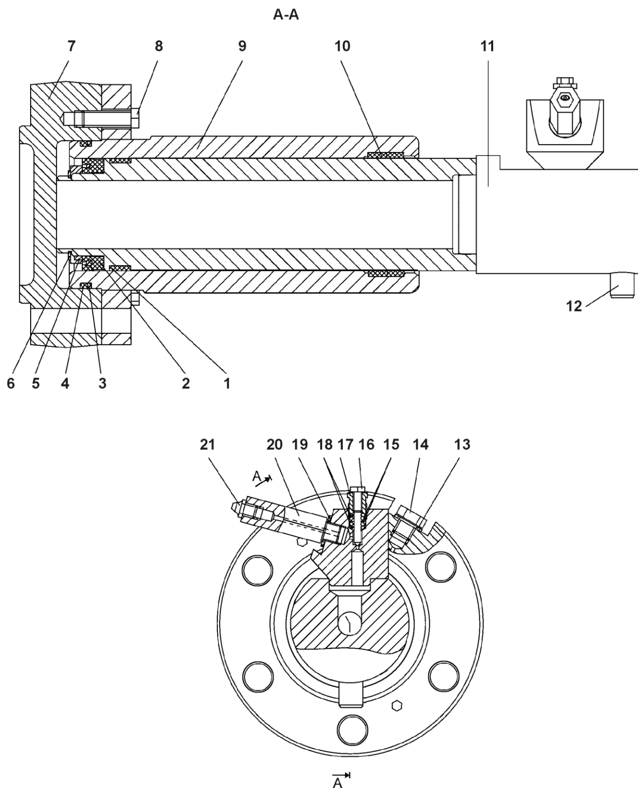
Рисунок 3.9 Механизм натяжения Figure 3.9 Track adjusting mechanism
