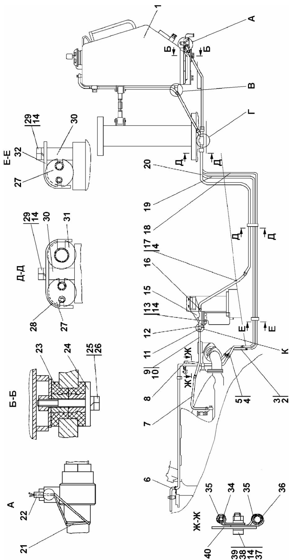
Рисунок 1.5 Установка топливного бака Figure 1.5 Fuel tank mounting
