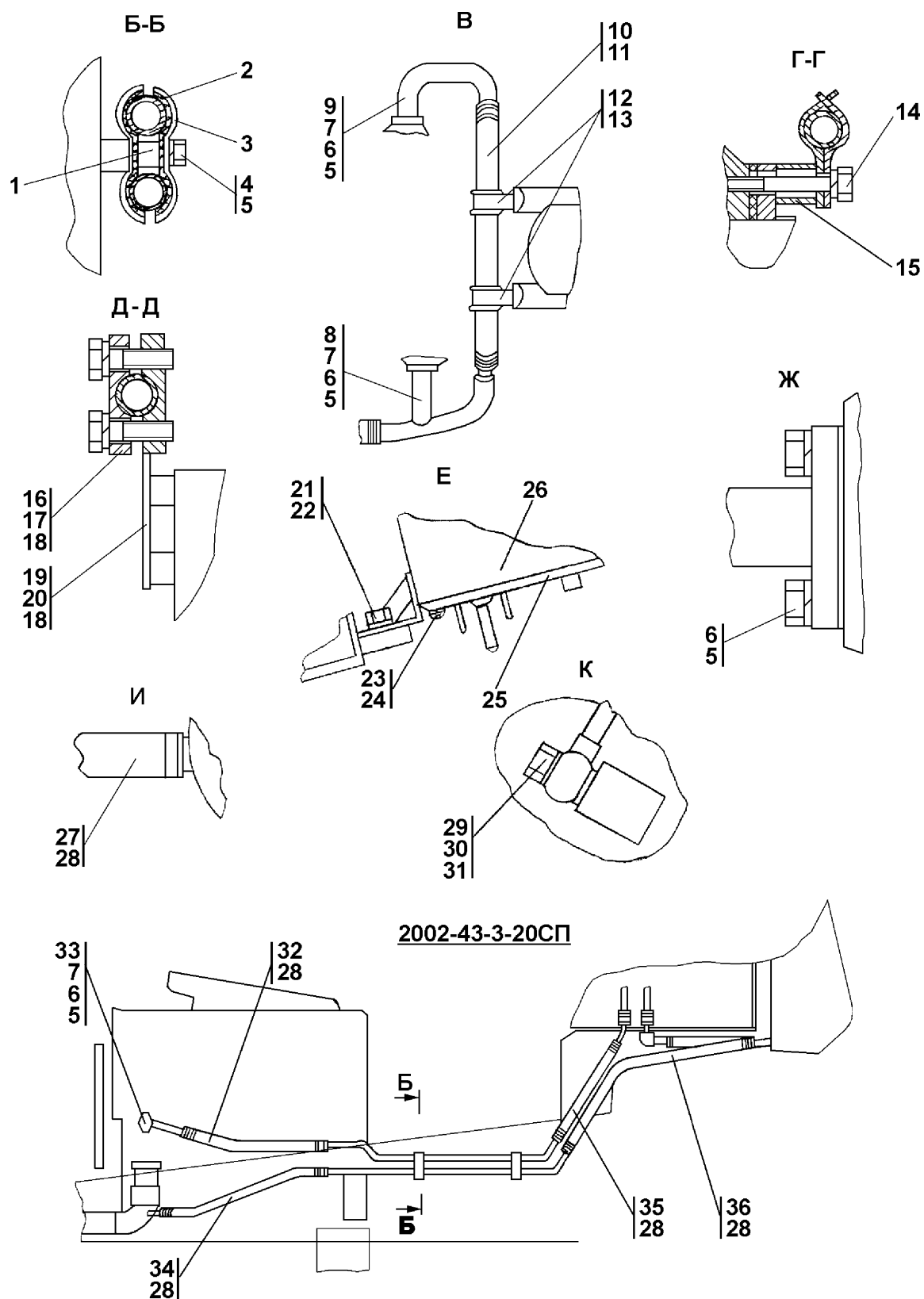
Рисунок 1.9 Установка системы подогрева Figure 1.9 Pre-heater system mounting
