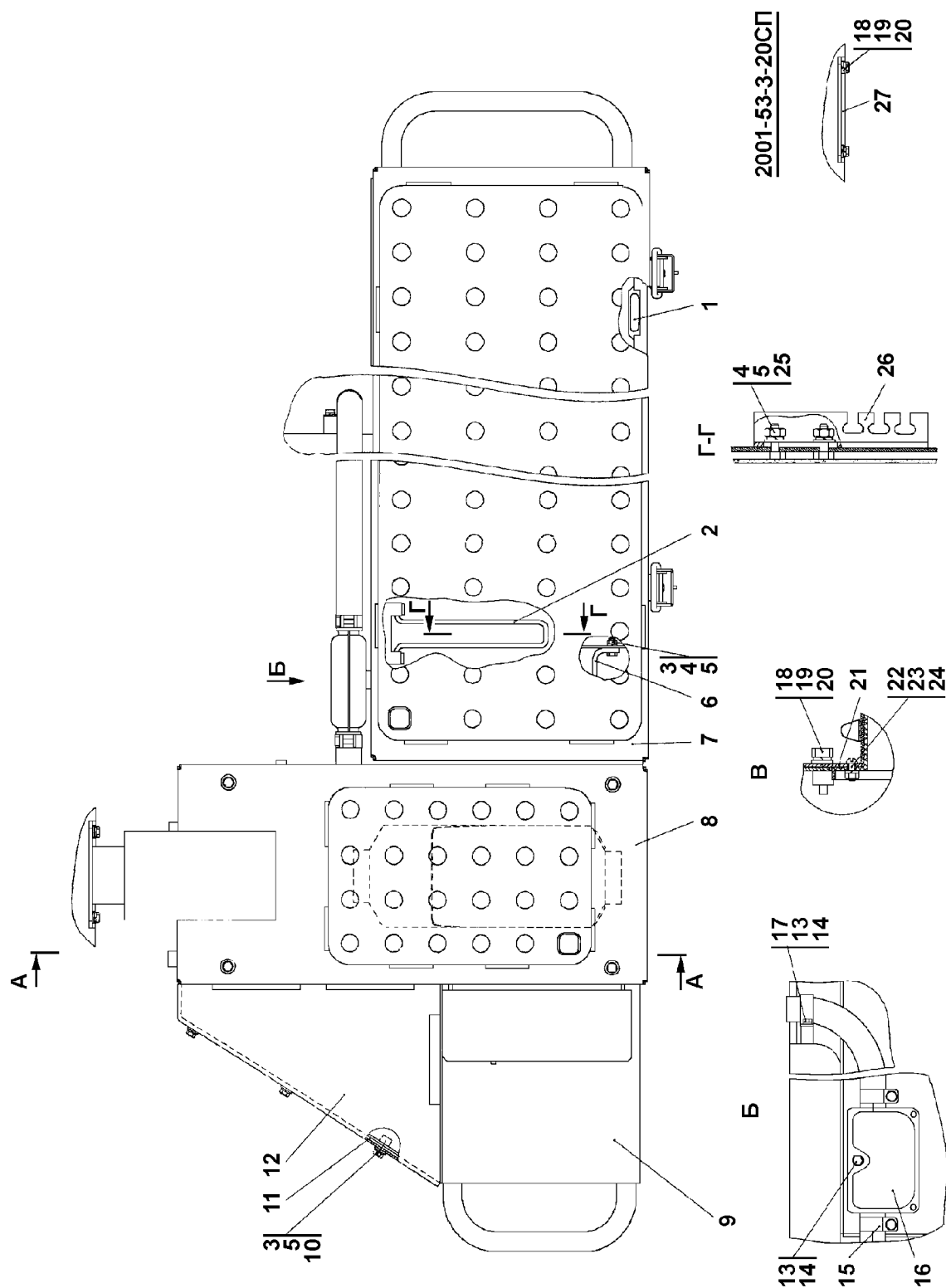
Рисунок 6.22 Установка независимого отопителя кабины Figure 6.6 Independent cab heater mounting
