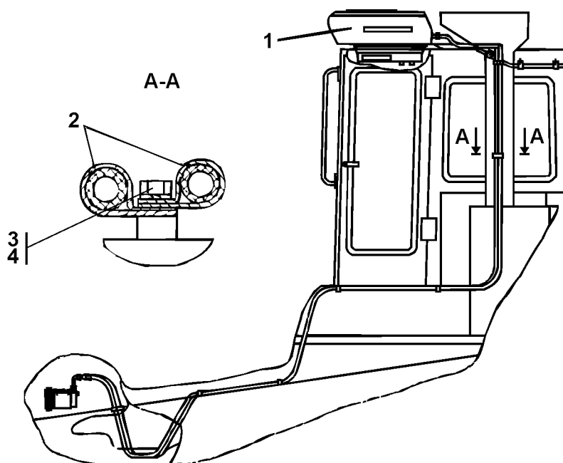
Рисунок 6.28 Установка кондиционера Figure 6.28 Conditioner mounting
