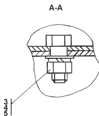
Рисунок 6.14 Установка сиденья Figure 6.14 Seat mounting
