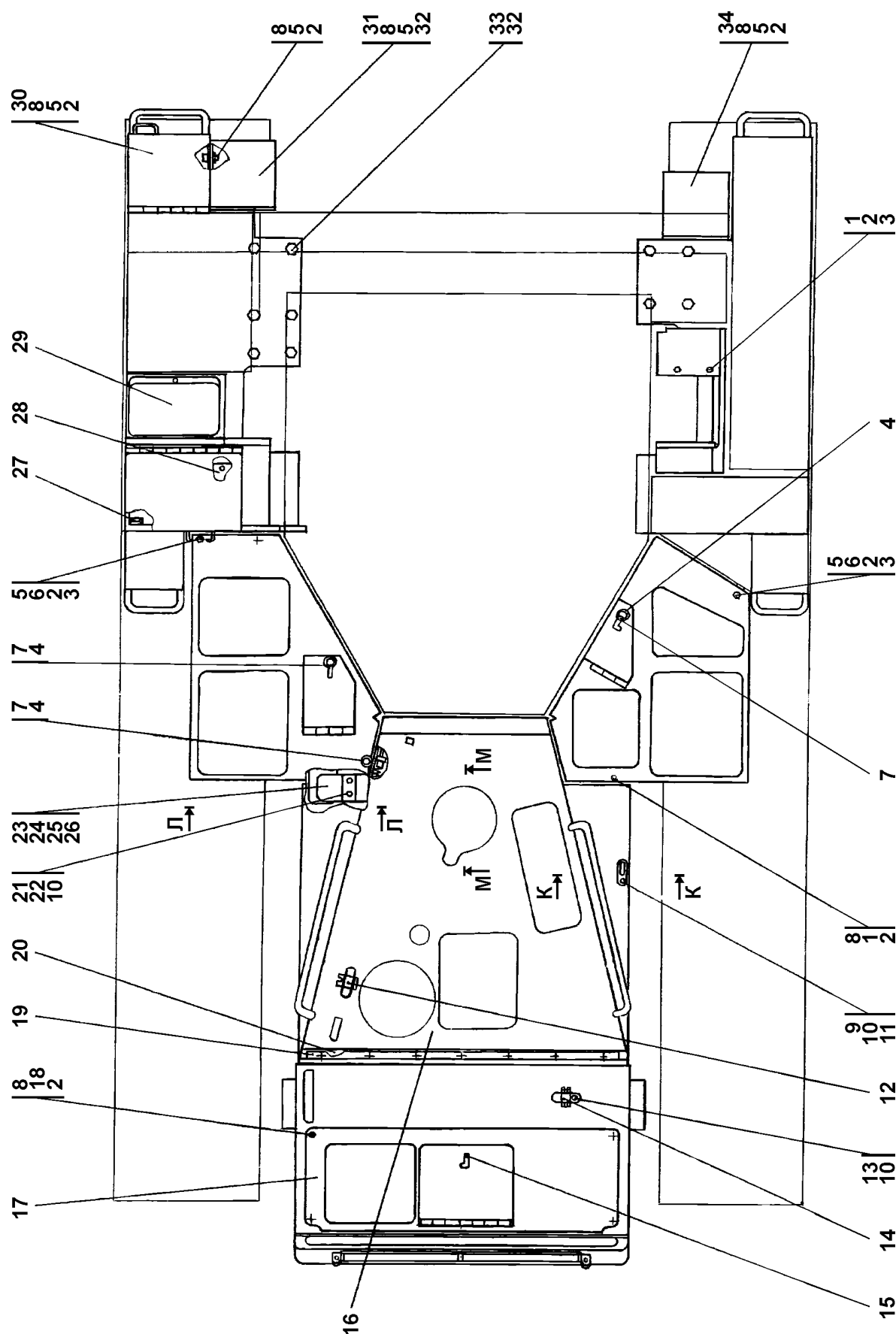
Рисунок 6.10 Облицовка Figure 6.10 Facing
