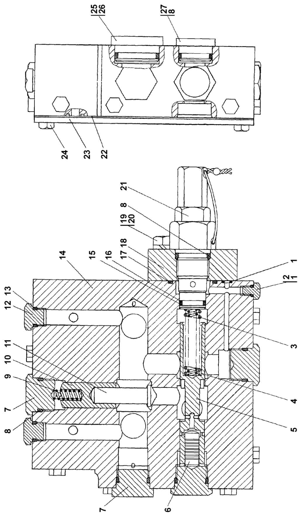
Рисунок 5.9 Клапан Figure 5.9 Valve
