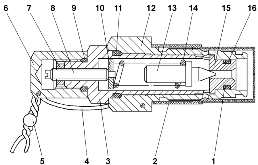
Рисунок 5.7 Клапан предохранительный Figure 5.7 Safety valve
