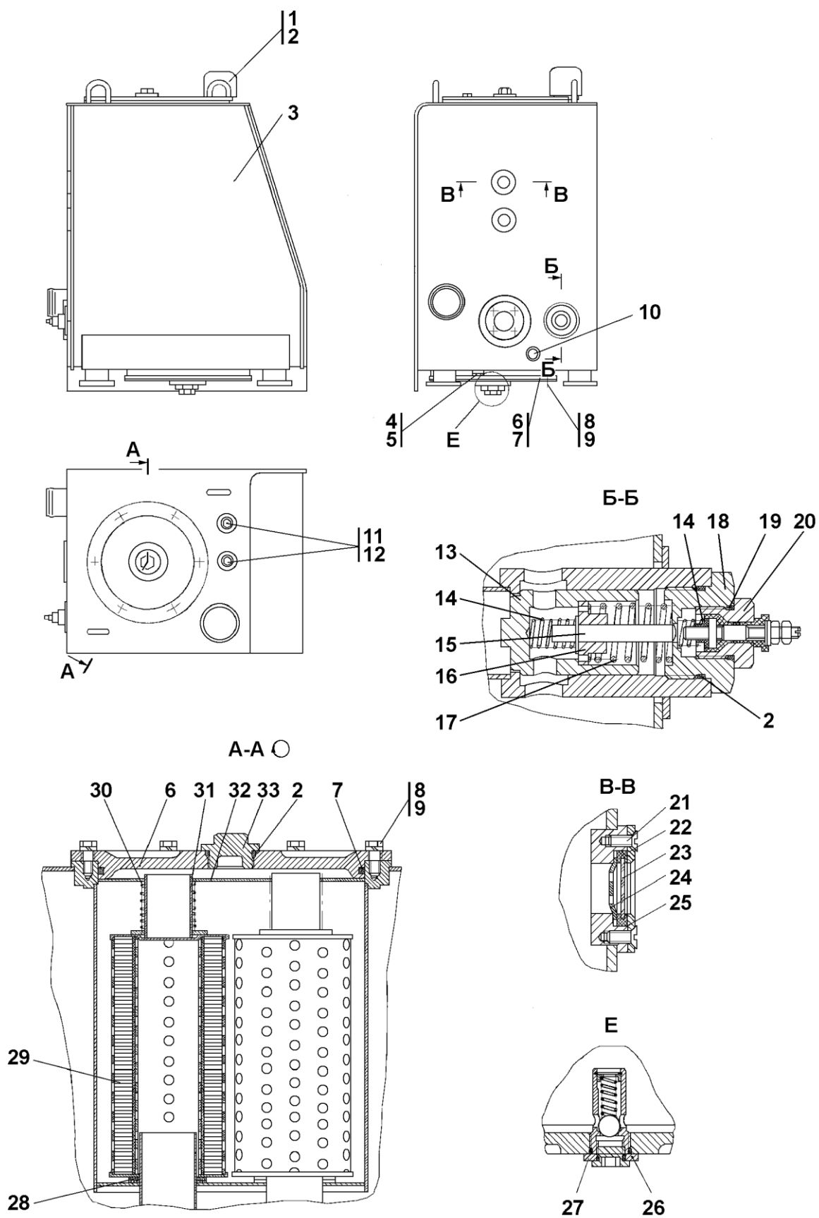
Рисунок 5.8 Бак гидросистемы Figure 5.8 Hydraulic system tank
