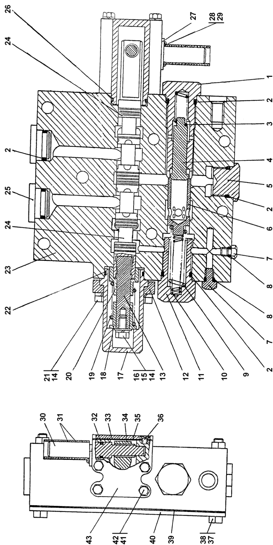
Рисунок 5.5 Распределитель Figure 5.5 Control valve
