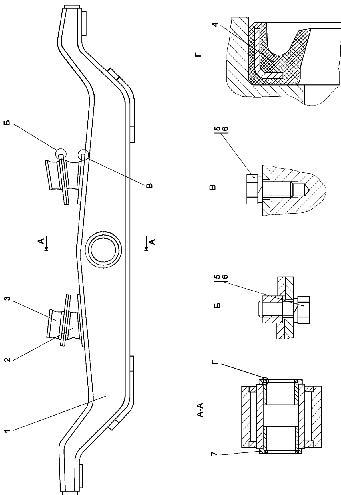
Рисунок 3.2 Балка Figurй2e 3.2 Beam
