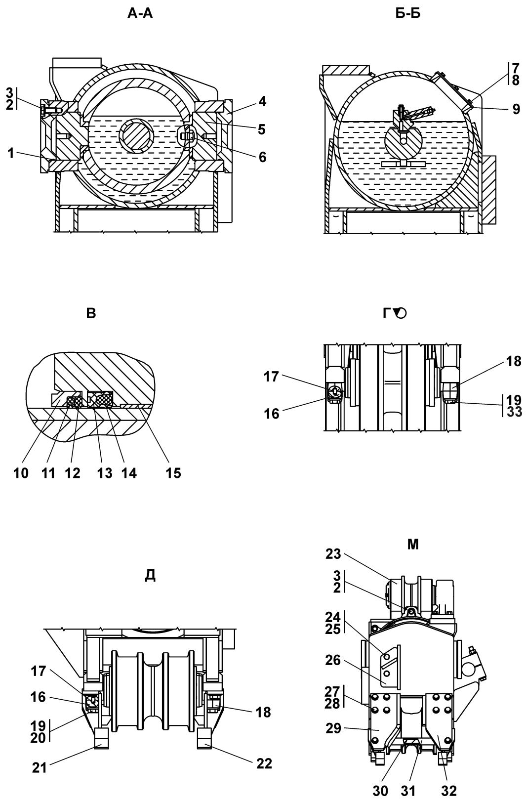
Рисунок 3.17 Тележка Figure 3.17 Bogie
