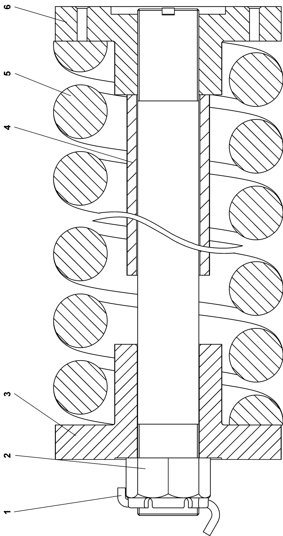
Рисунок 3.20 Механизм сдавания Figure 3.20 Track-release mechanism
