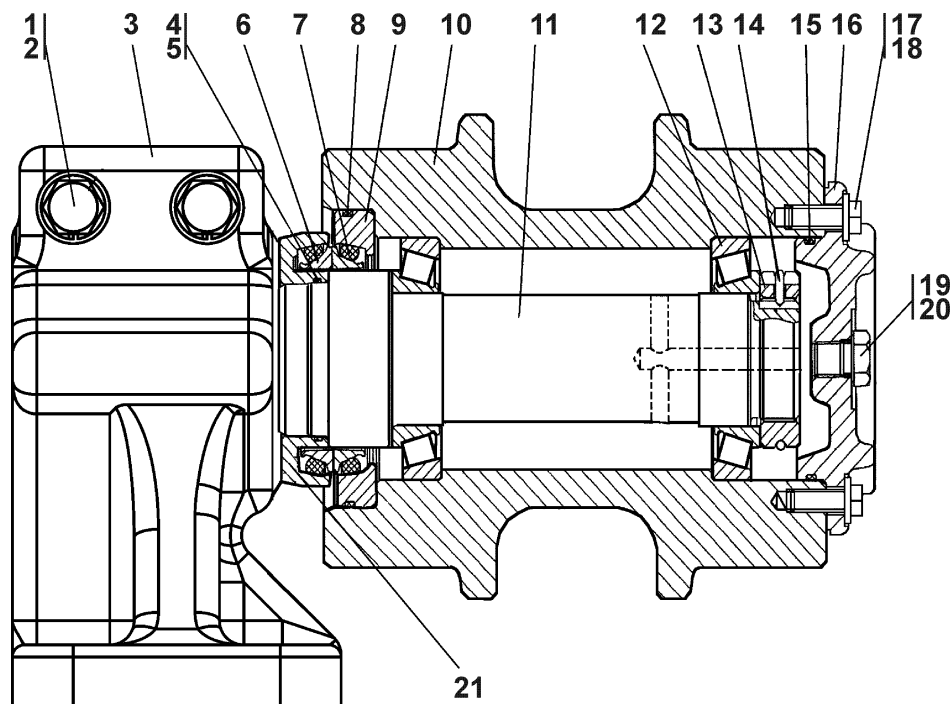
Рисунок 3.18 Каток поддерживающий Figure 3.18 Support roller
