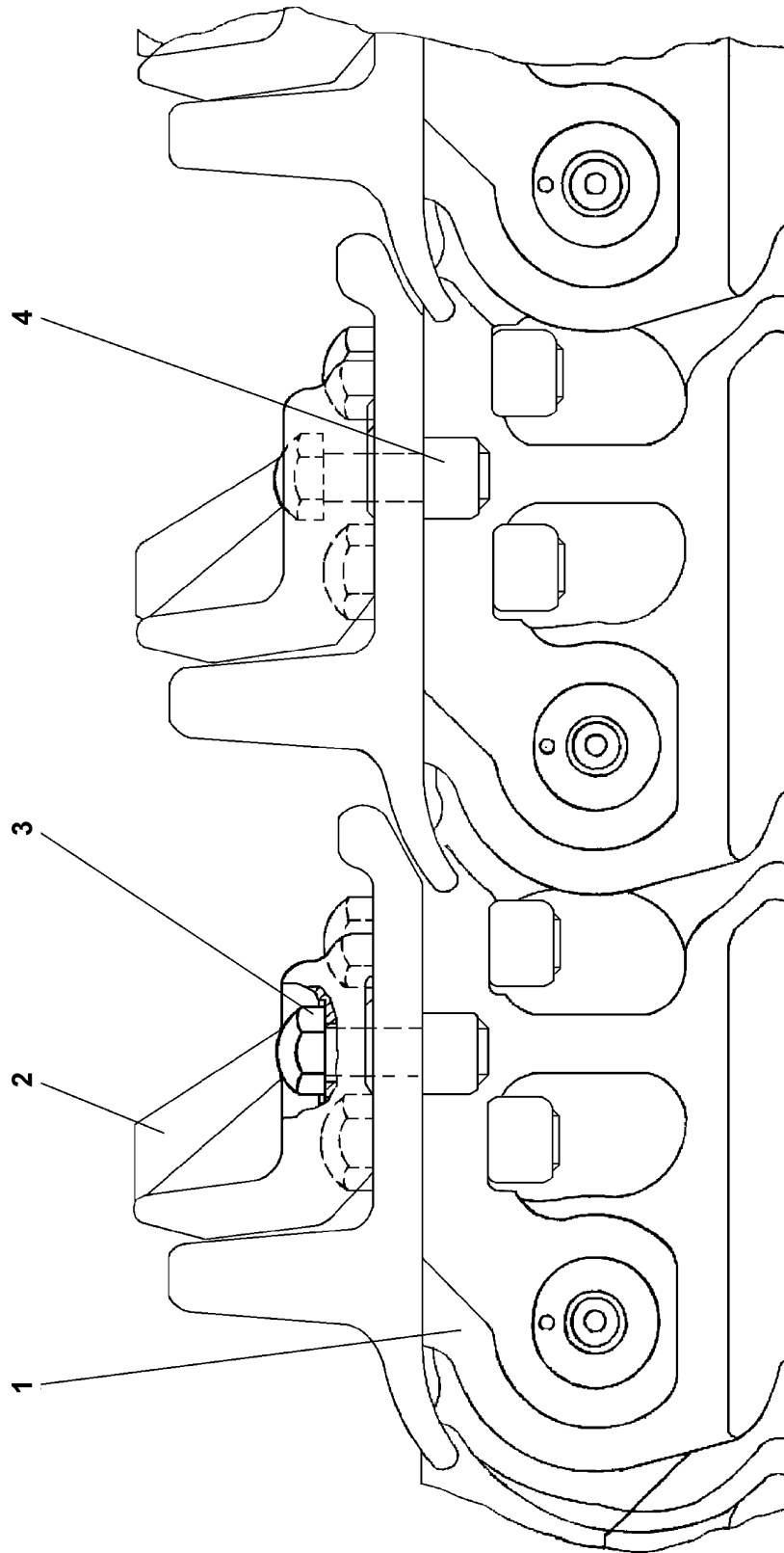
Рисунок 3.23 Установка ледоходных шпор на гусеницу Figure 3.23 Ice moving spurs mounting on the track
