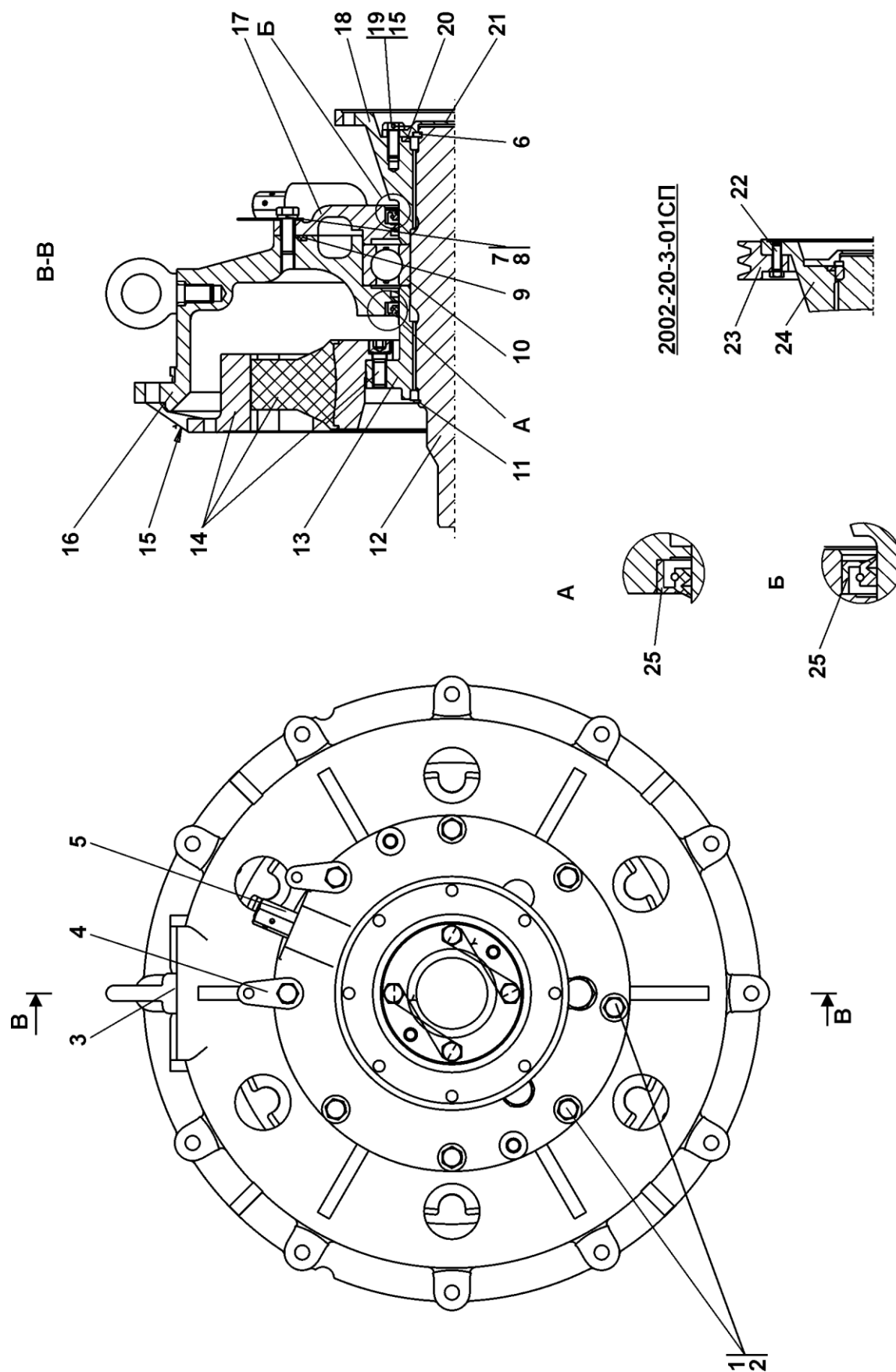
Рисунок 4.26 Муфта упругая Figure 4.26 Elastic coupling
