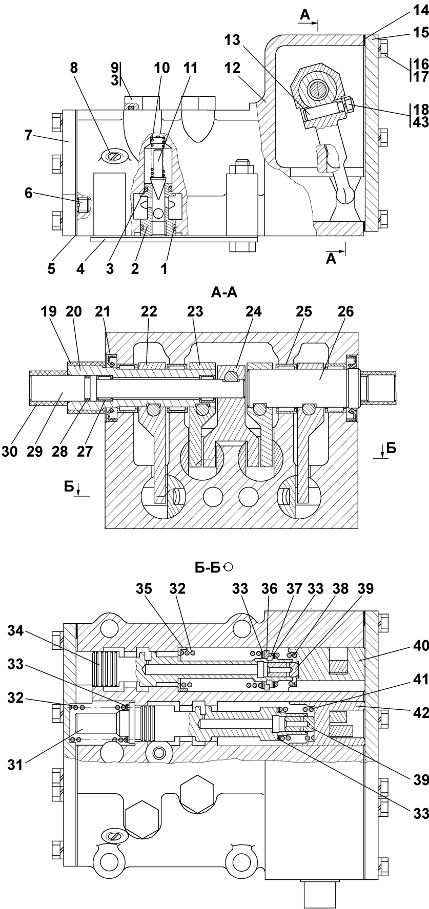
Рисунок 4.21 Блок управления Figure 4.21 Control unit
