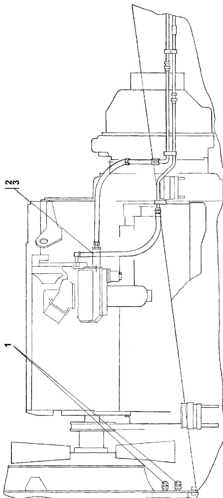
Рисунок 1.6 Установка топливного бака Figure 1.6 Fuel tank mounting
