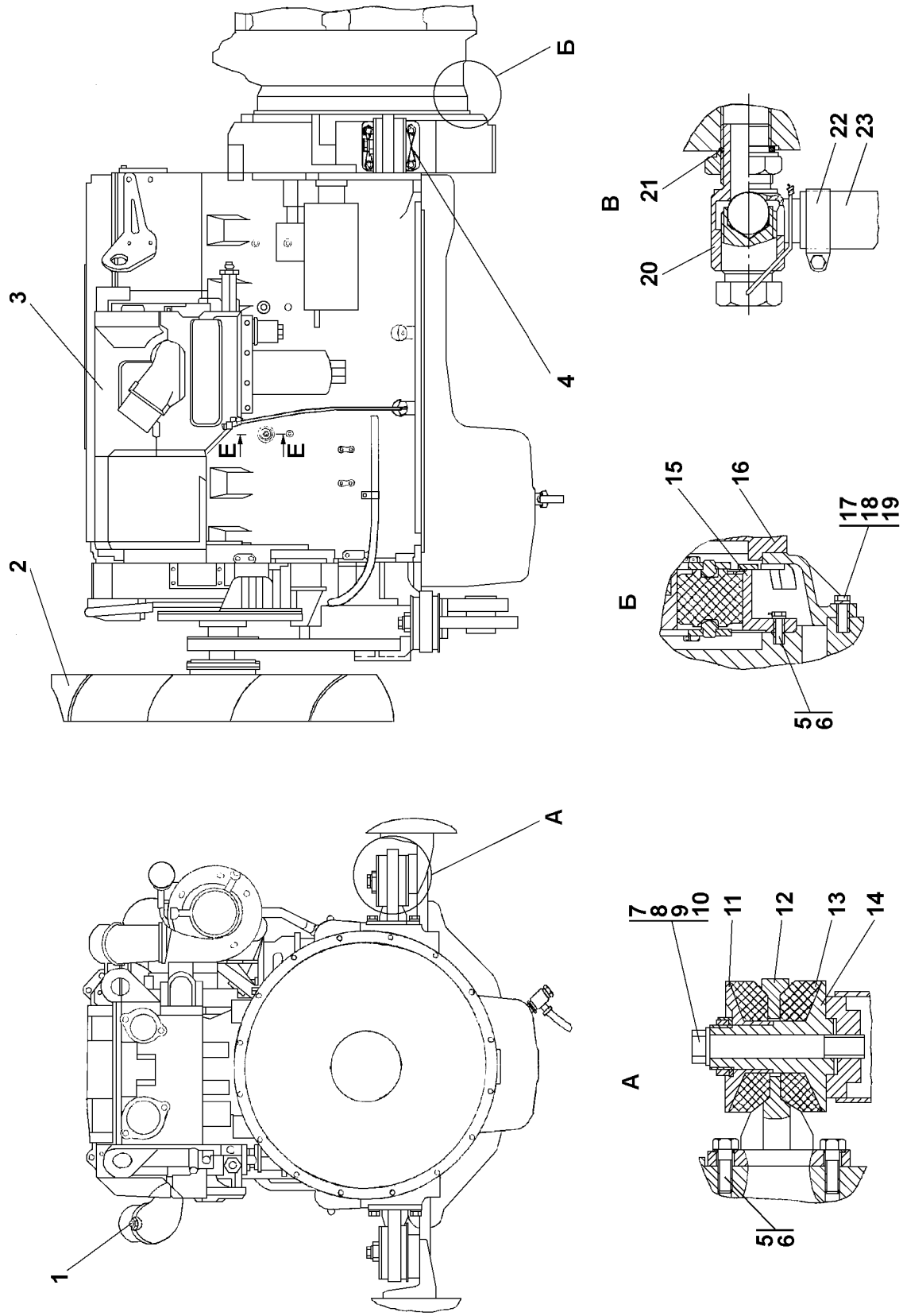
Рисунок 1.1 Установка двигателя QSX15-C440 «Cummins» Figure 1.1 QSX15-C440 «Cummins» Engine mounting
