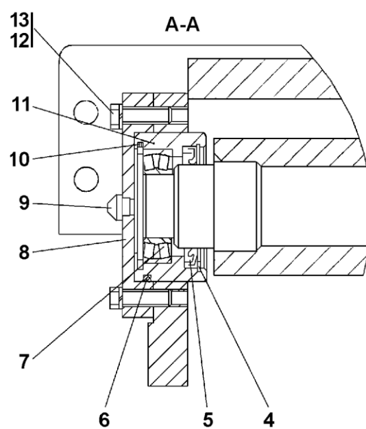
Рисунок 7.22 Установка роликов Figure 7.22 Roller mounting
