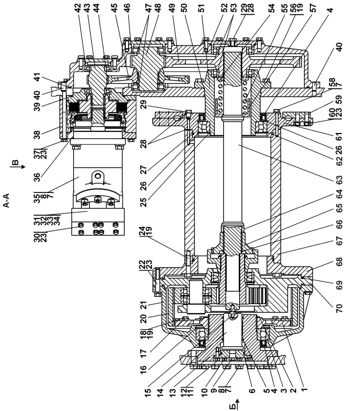
Рисунок 7.21 Лебедка Figure 7.21 Winch
