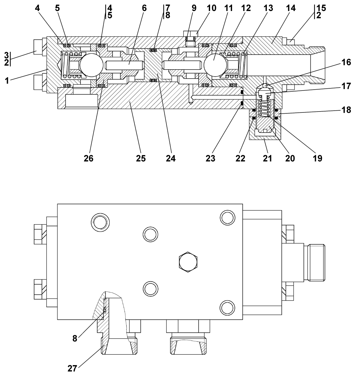
Рисунок 7.12 Гидрозамок Figure 7.12 Pilot controlled check valve
