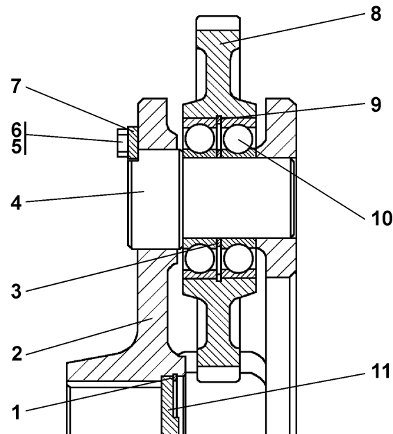
Рисунок 7.34 Водило Figure 7.34 Carrier
