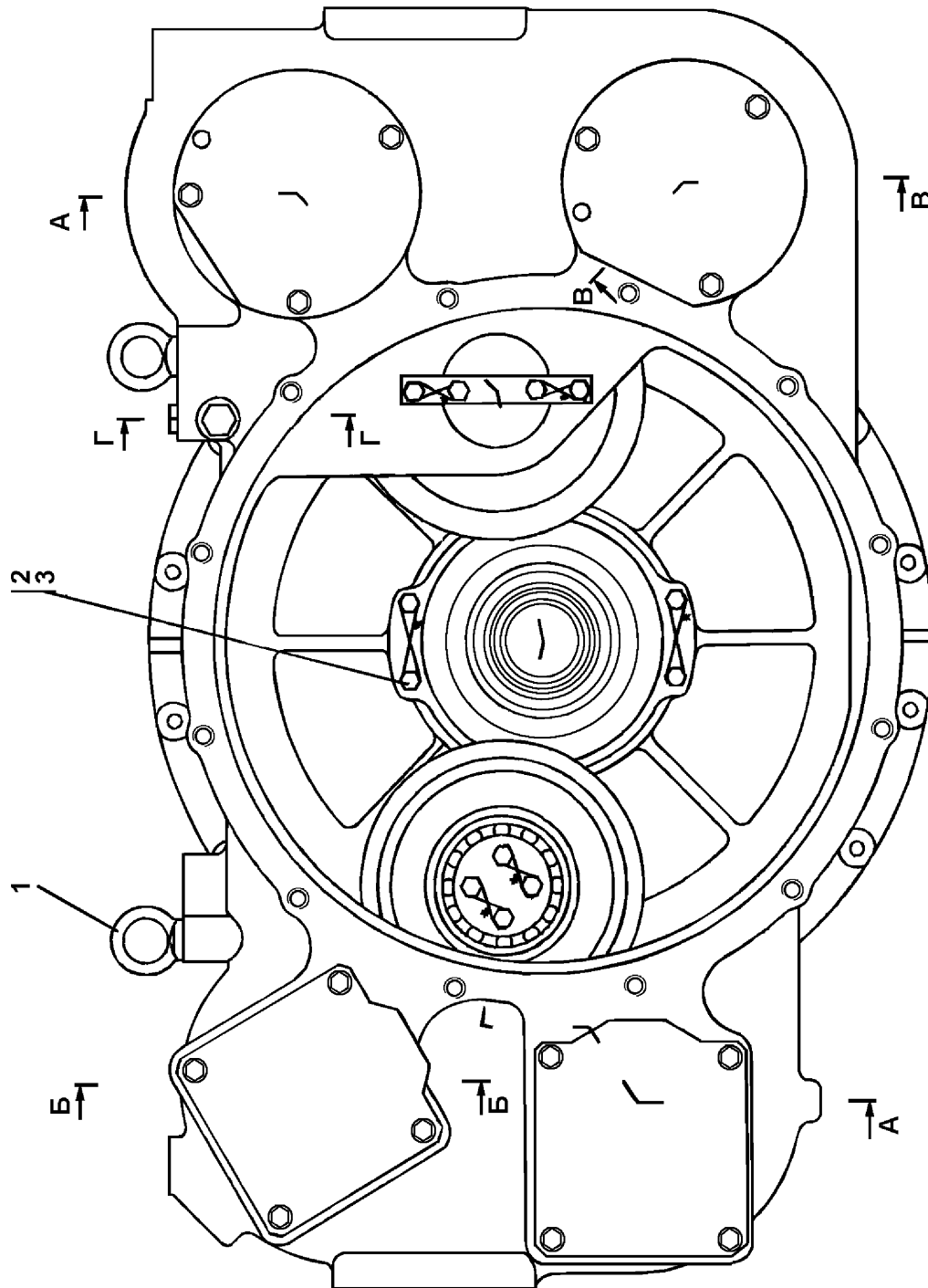
Рисунок 4.22 Редуктор привода насосов Figure 4.22 Pump drive reduction gear
