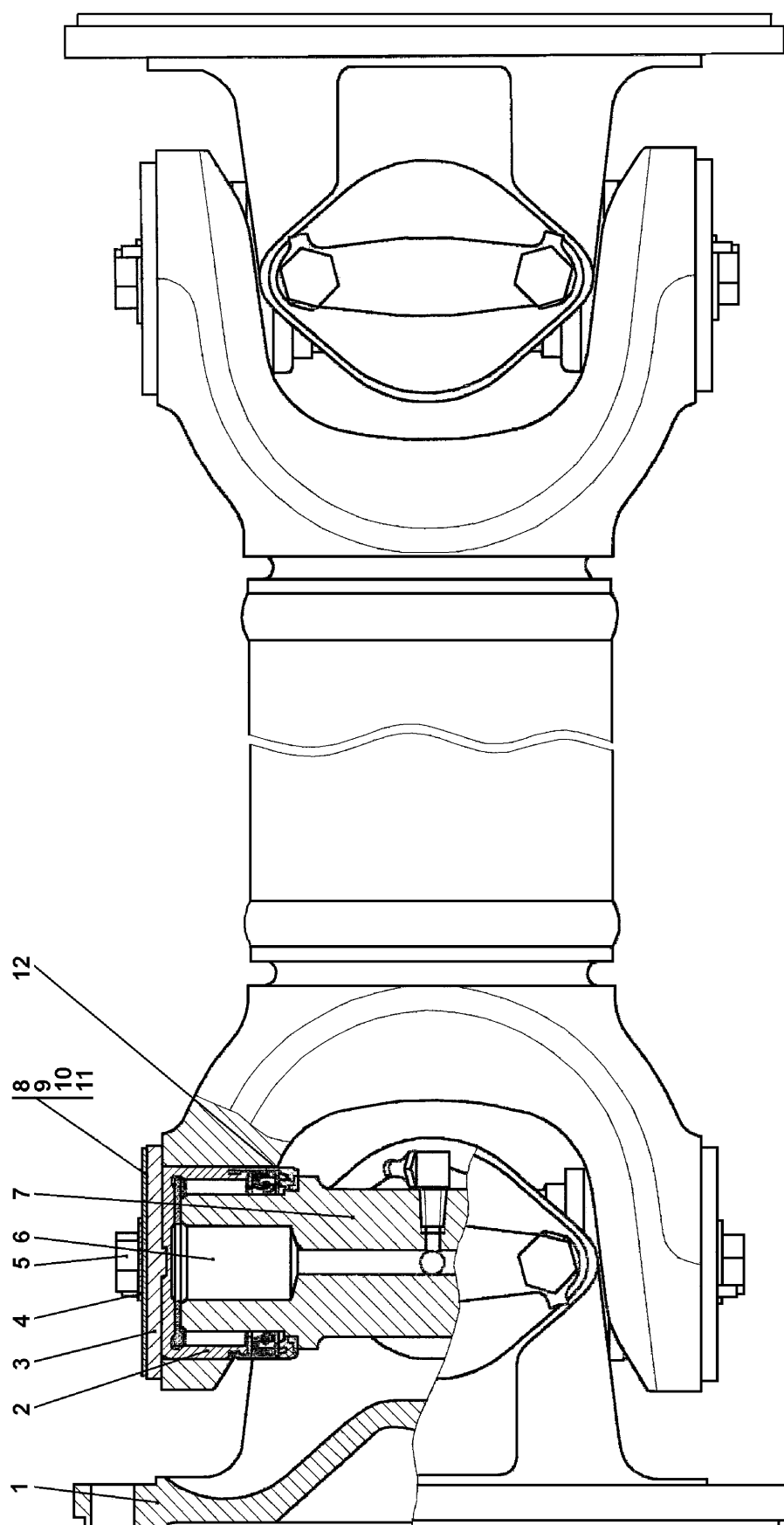
Рисунок 4.26 Вал карданный Figure 4.26 Cardan shaft
