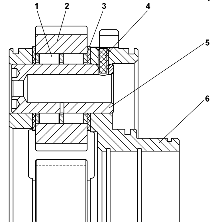
Рисунок 4.11 Водило Figure 4.11 Carrier
