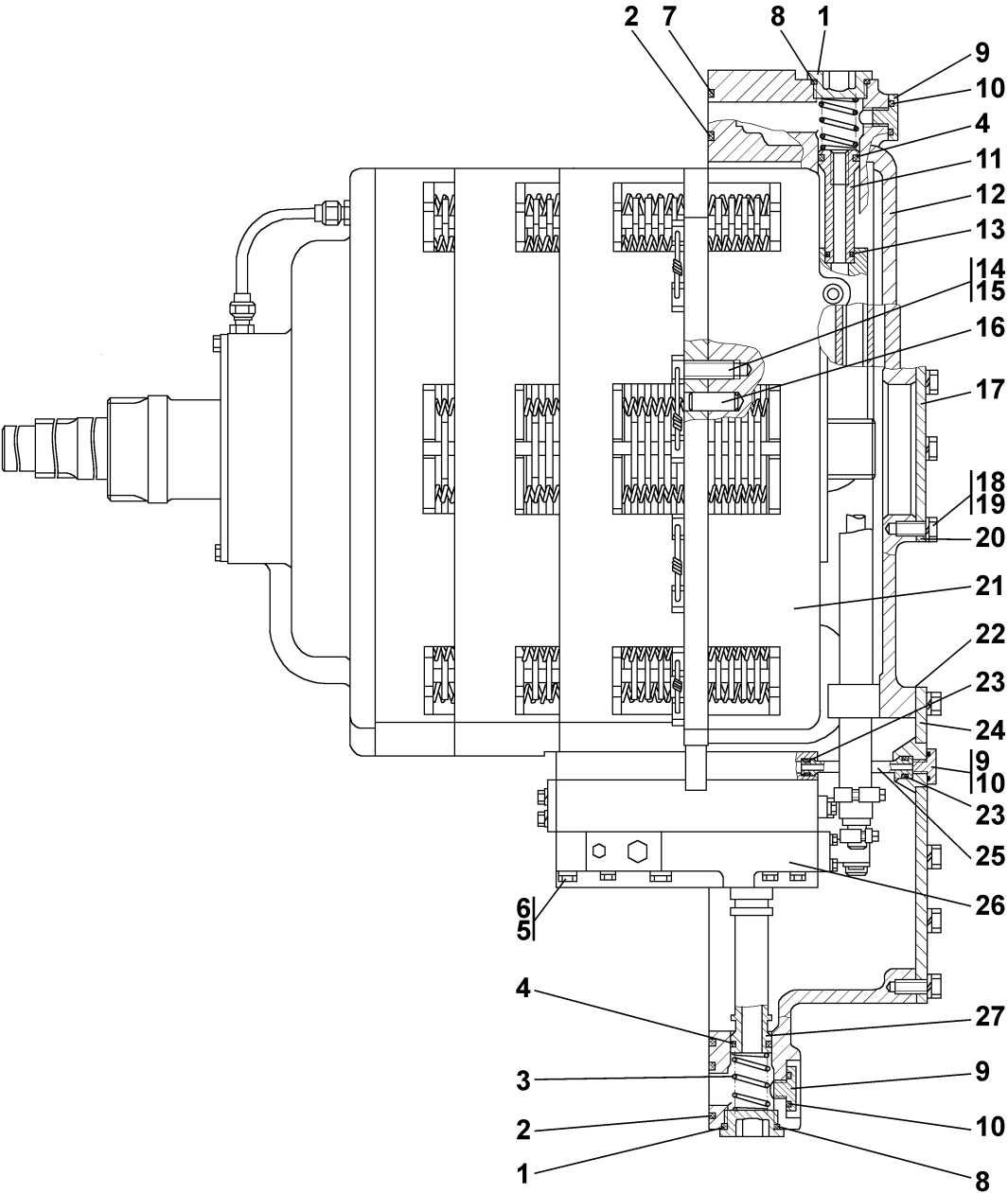
Рисунок 4.7 Коробка передач с системой гидроуправления Figure 4.7 Gearbox with hydraulic control system
