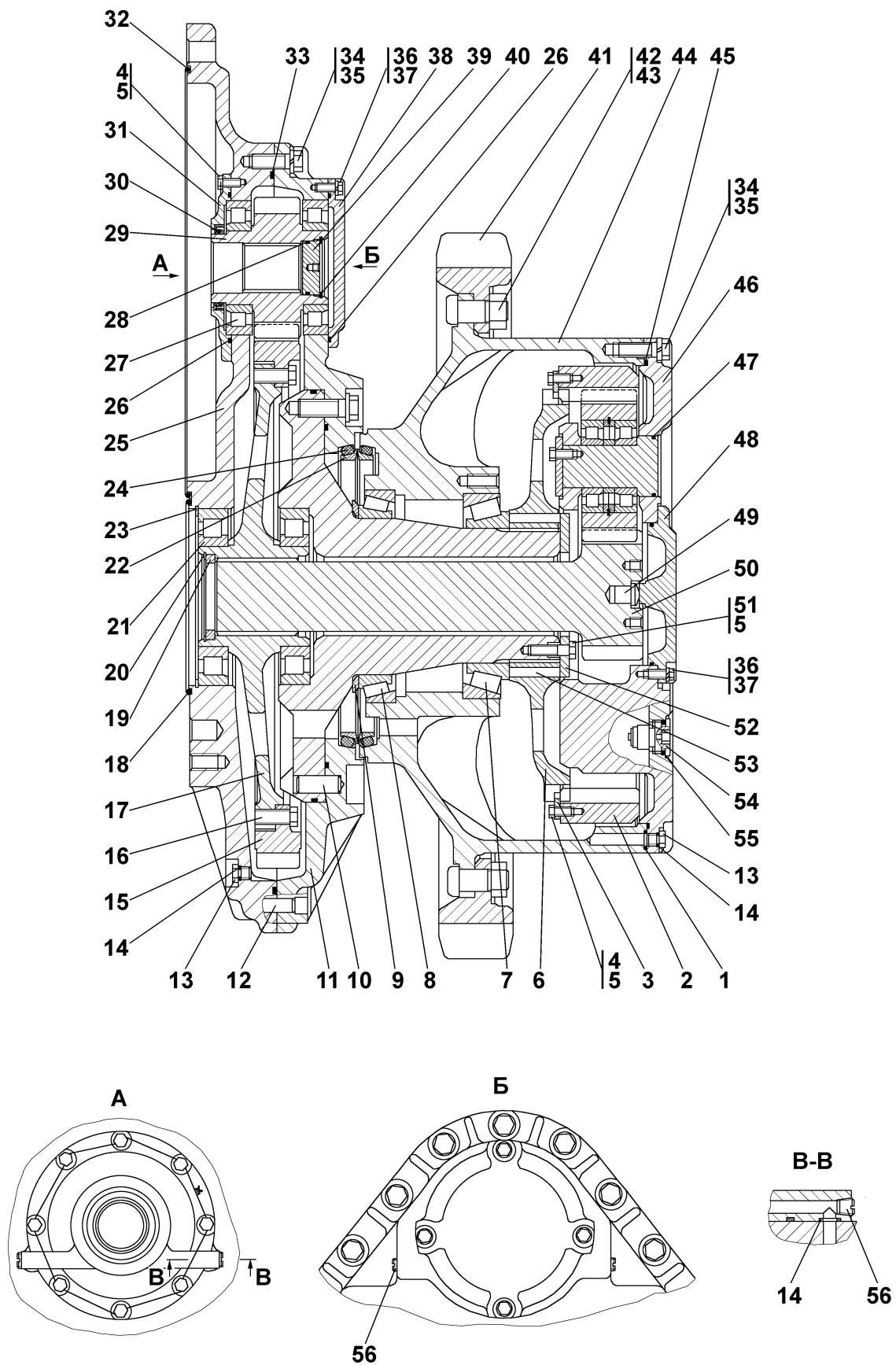
Рисунок 4.25 Передача бортовая Figure 4.25 Final drive
