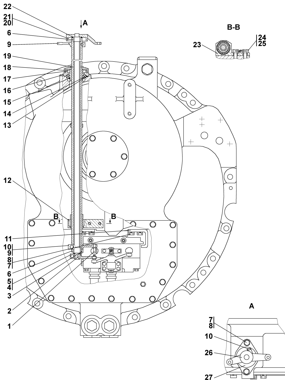
Рисунок 4.6 Коробка передач с системой гидроуправления Figure 4.6 Gearbox with hydraulic control system
