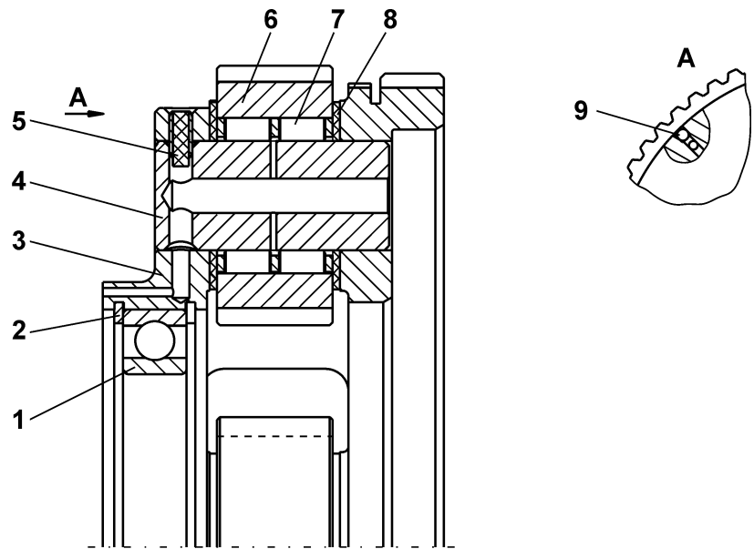
Рисунок 4.10 Водило Figure 4.10 Carrier
