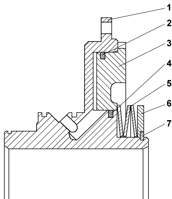
Рисунок 4.9 Бустер Figure 4.9 Booster
