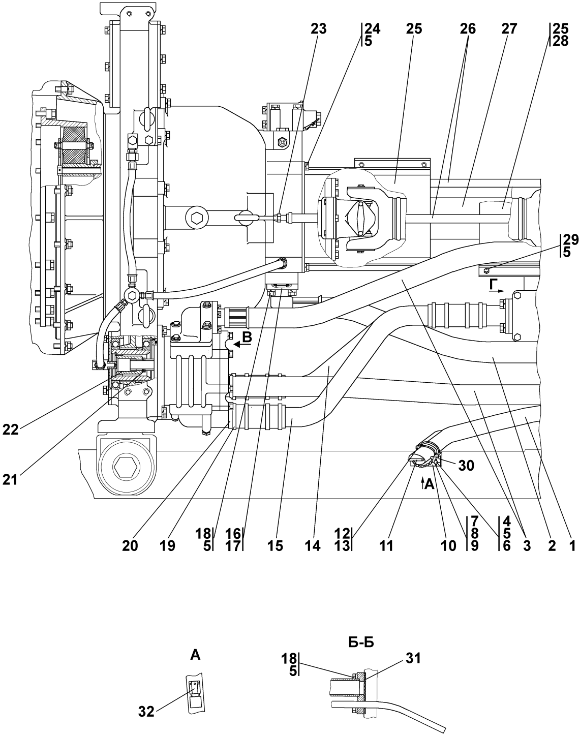
Рисунок 4.1 Установка трансмиссии Figure 4.1 Transmission mounting
