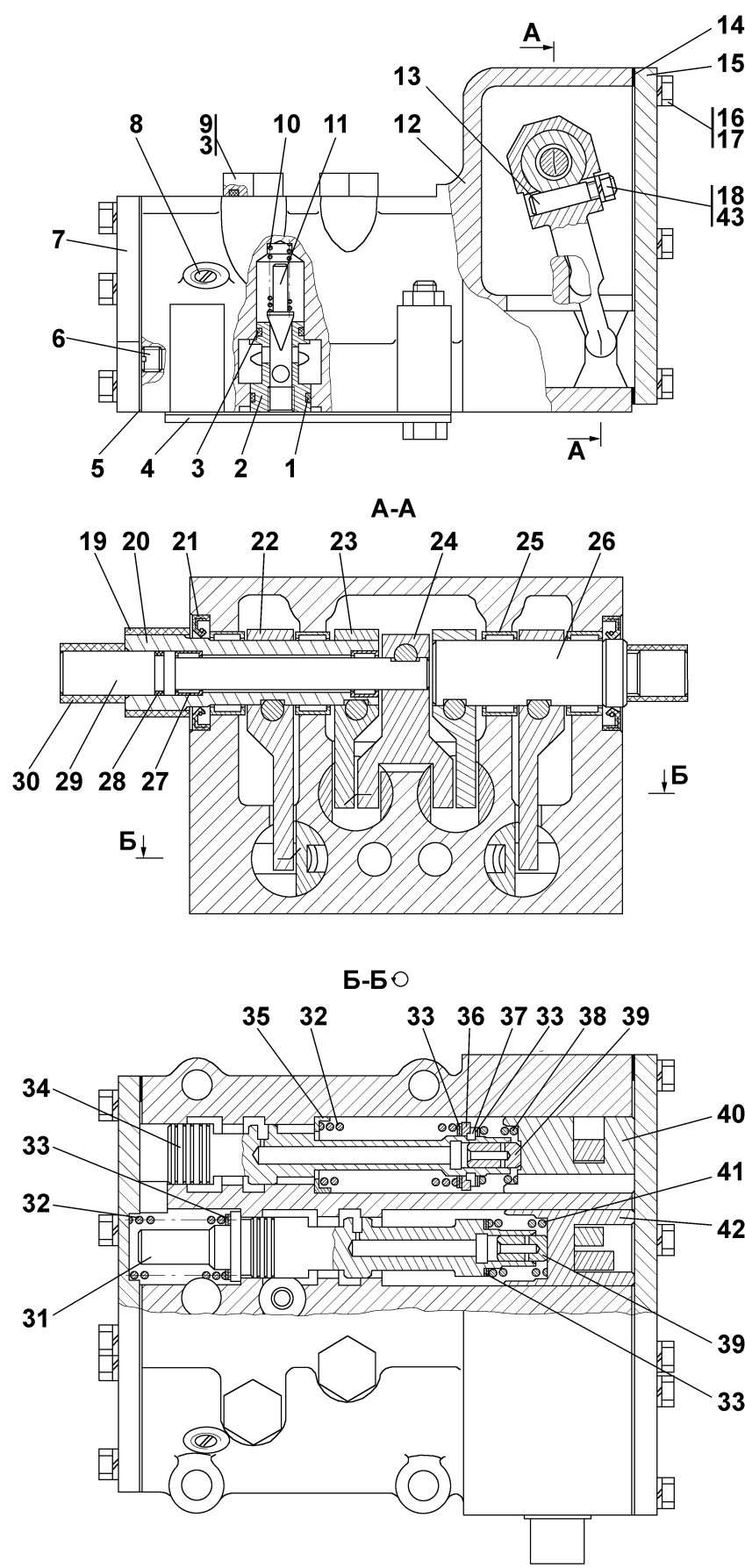
Рисунок 4.18 Блок управления Figure 4.18 Control unit
