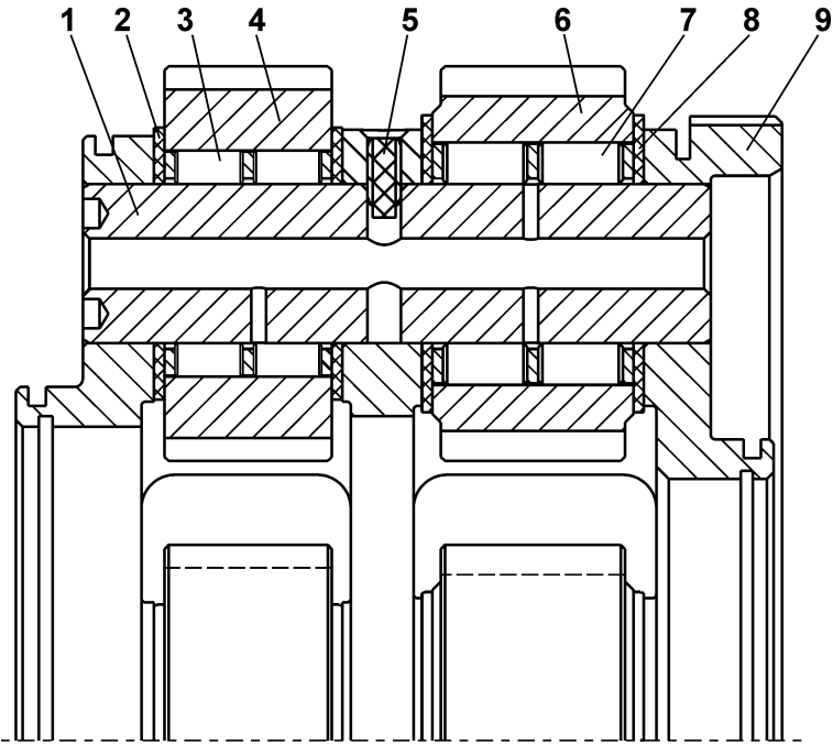
Рисунок 4.12 Водило Figure 4.12 Carrier
