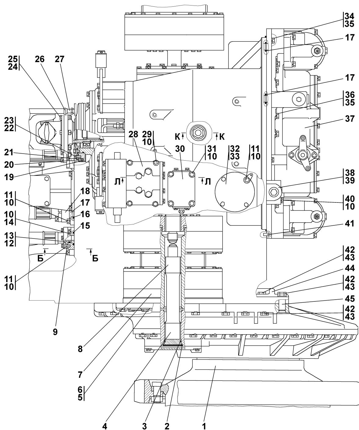
Рисунок 4.2 Установка трансмиссии Figure 4.2 Transmission mounting
