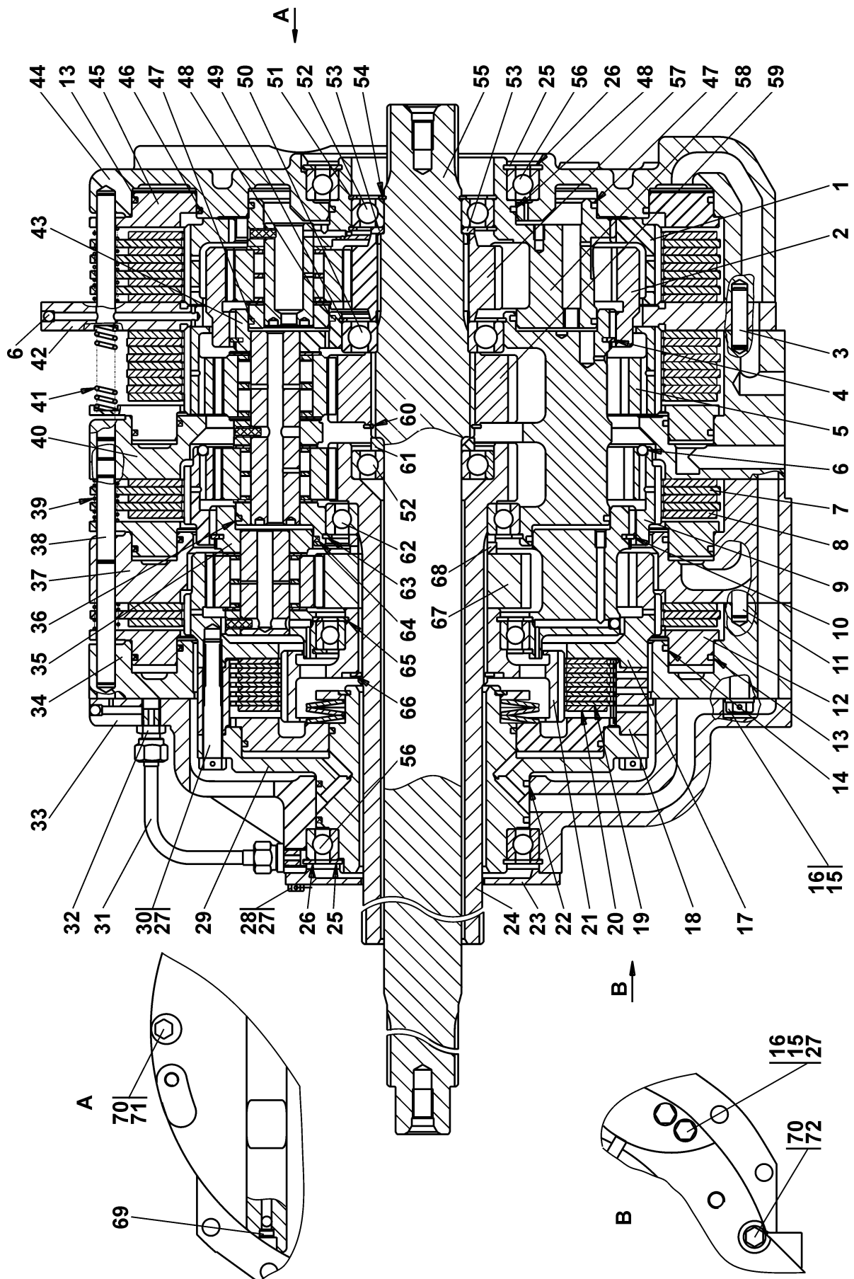
Рисунок 4.8 Коробка передач планетарная Figure 4.8 Planetary gearbox
