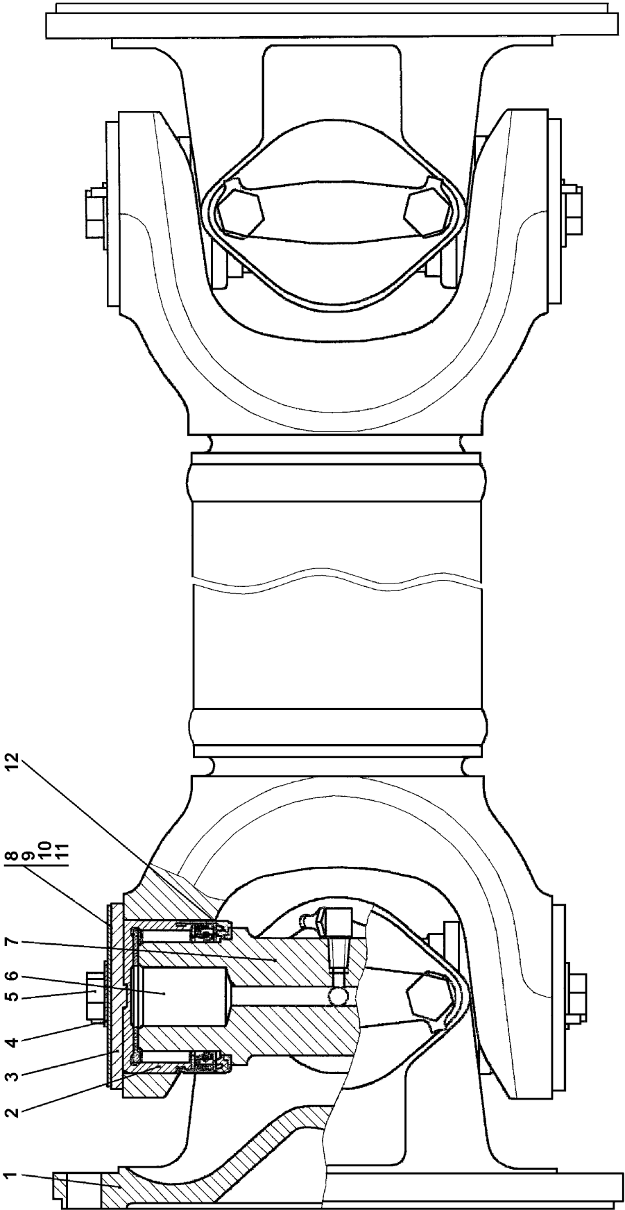
Рисунок 4.26 Вал карданный Figure 4.26 Cardan shaft
