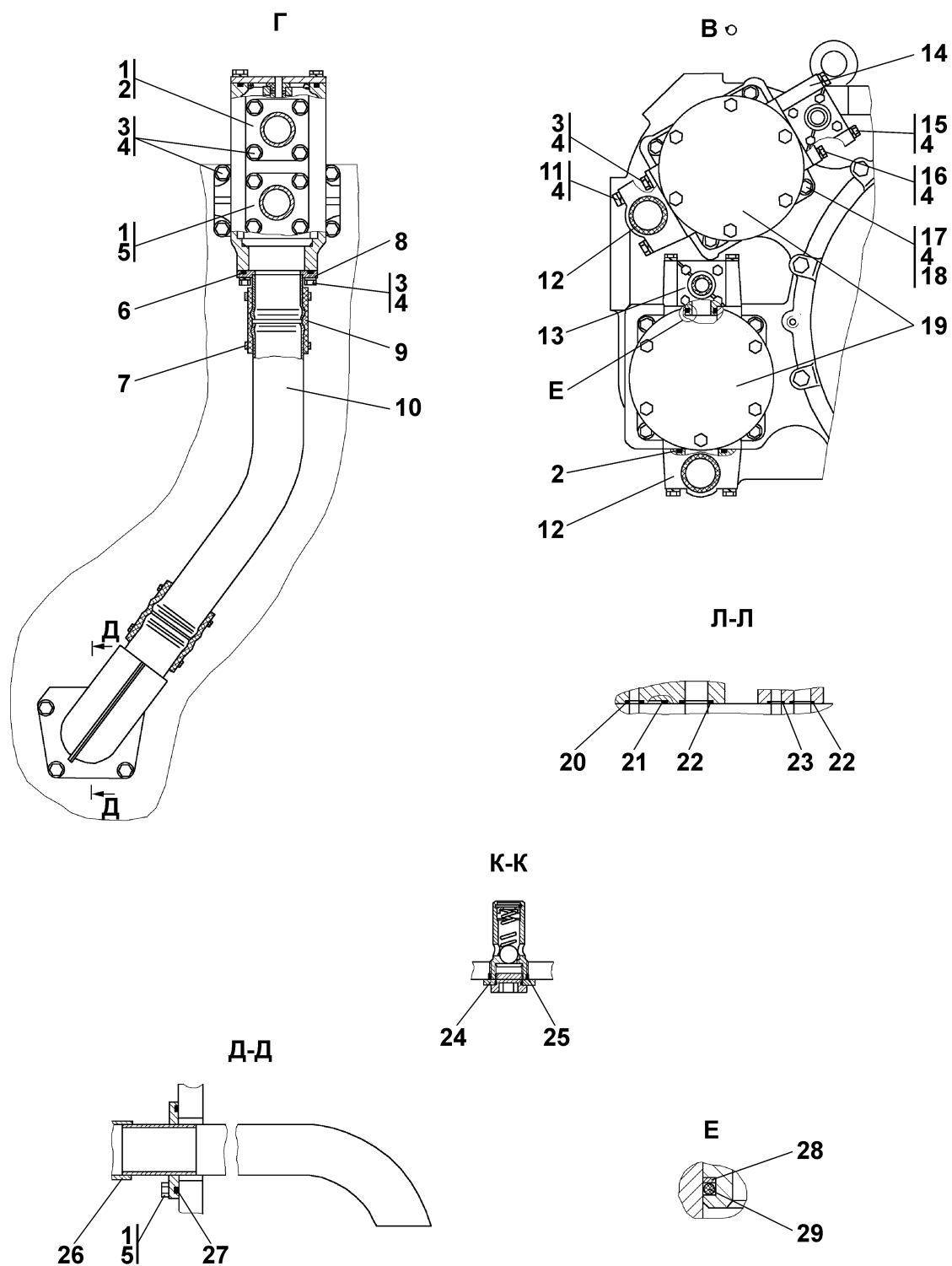
Рисунок 4.3 Установка трансмиссии Figure 4.3 Transmission mounting
