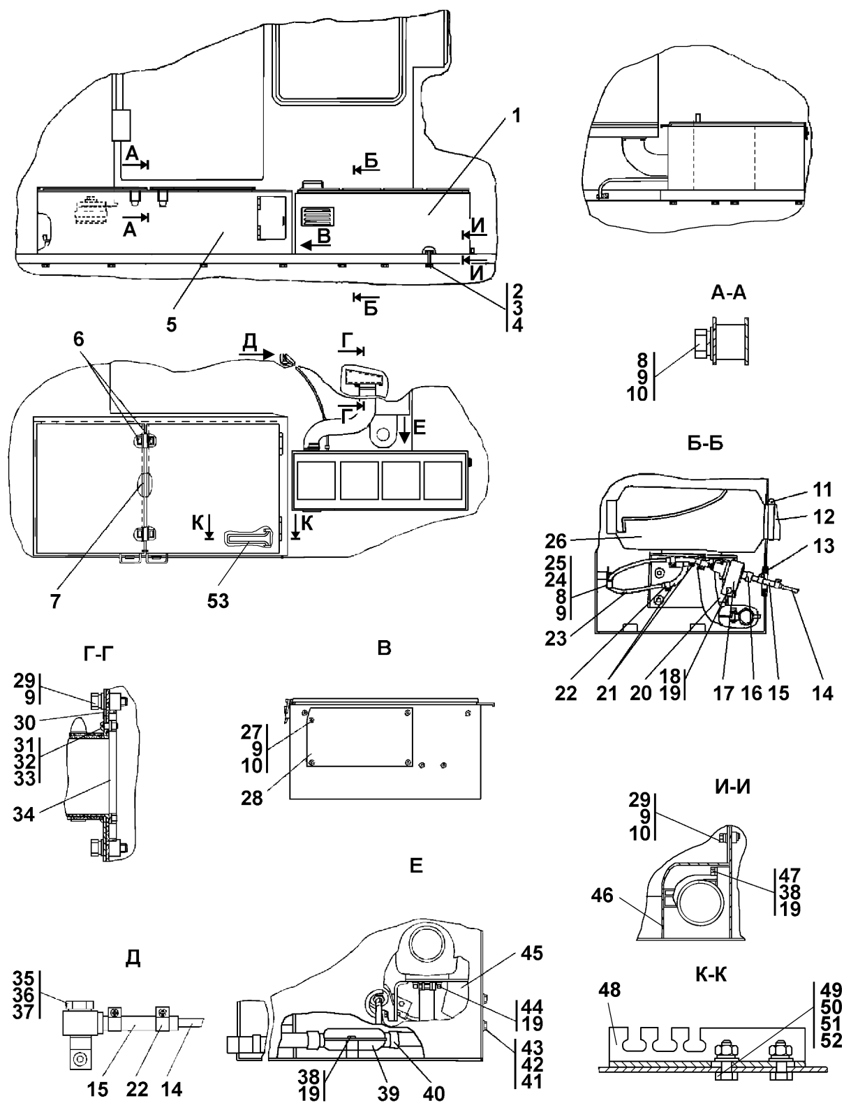
Рисунок 6.17 Система отопления и вентиляции кабины Figure 6.17 Cab heating and ventilation system
