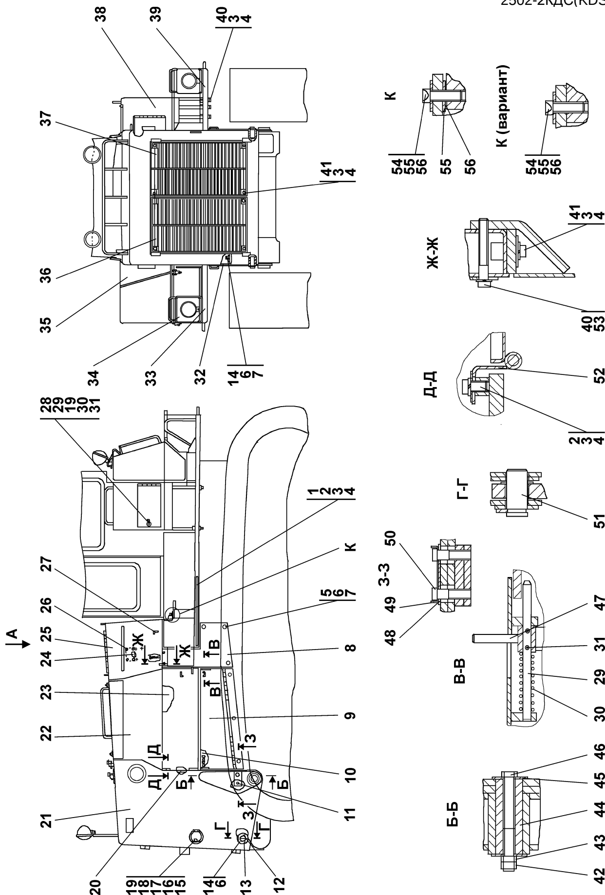
Рисунок 6.18 Облицовка Figure 6.18 Facing
