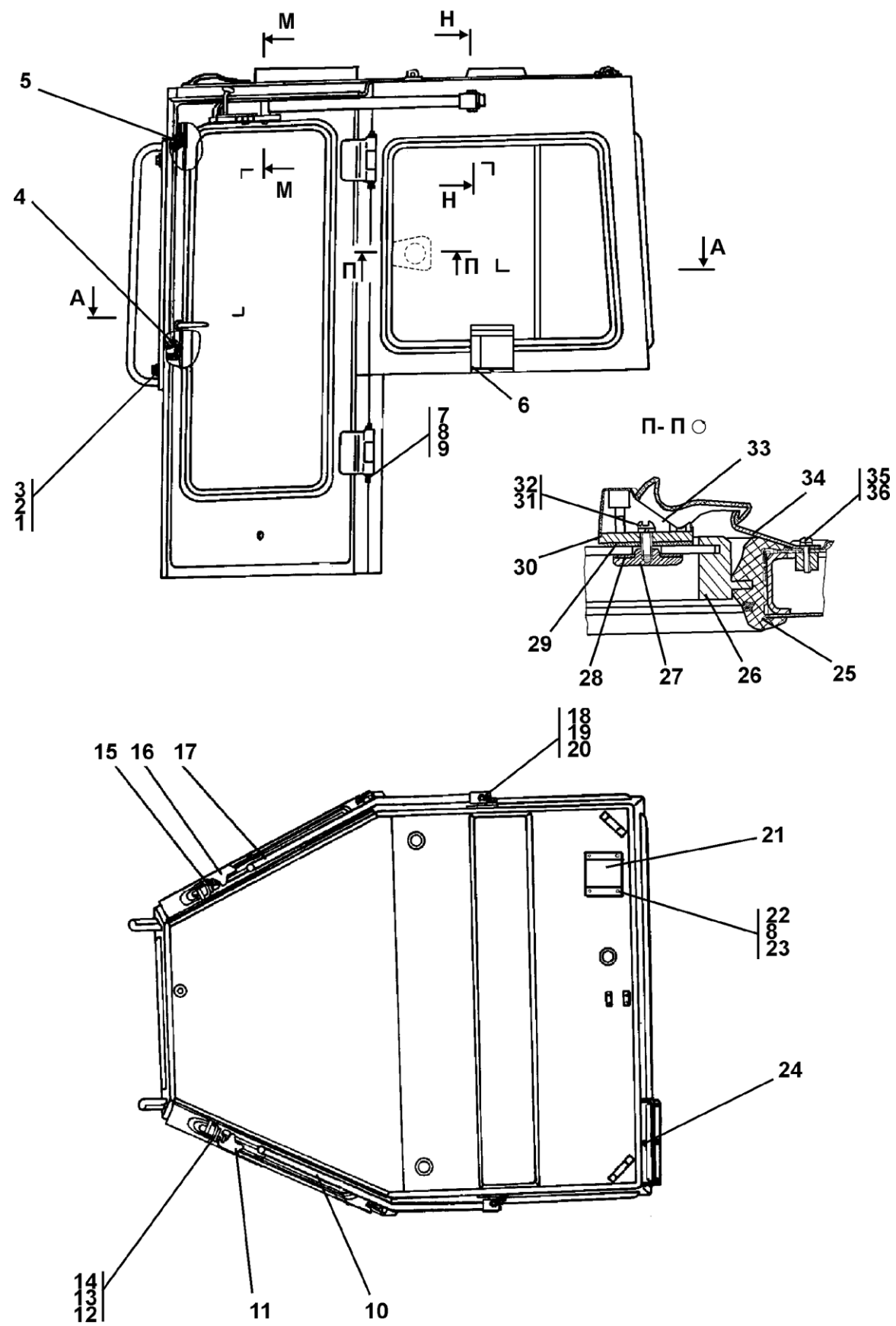
Рисунок 6.21 Кабина Figure 6.21 Cab
