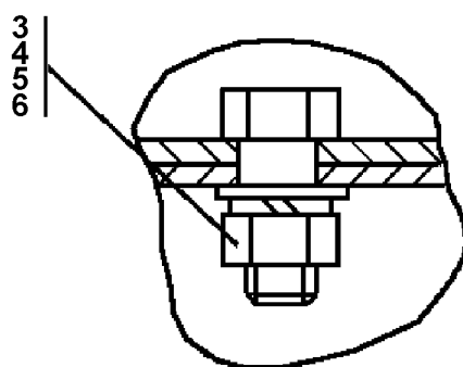
Рисунок 6.14 Установка сиденья Figure 6.14 Seat mounting
