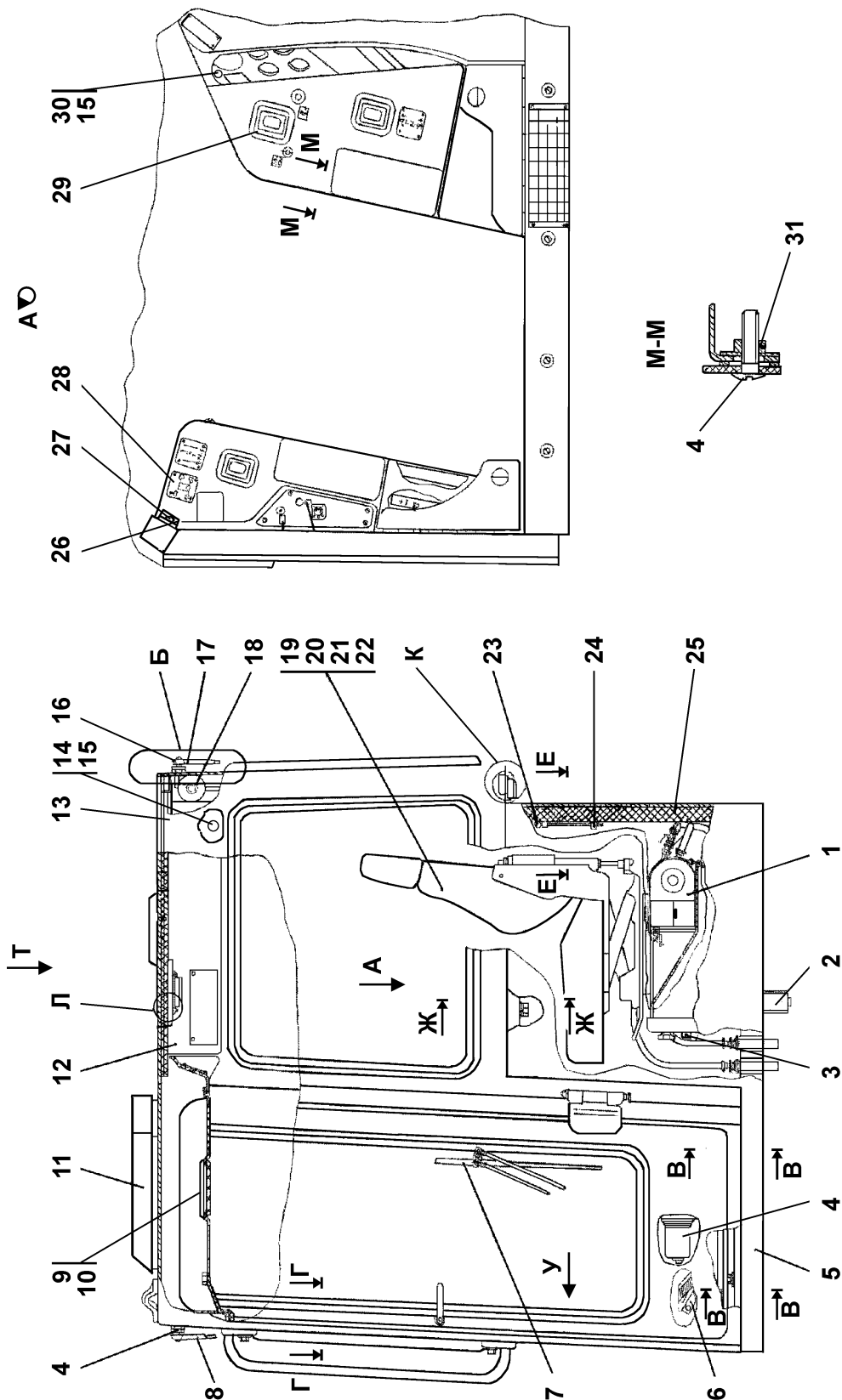
Рисунок 6.5 Кабина Figure 6.5 Cab
