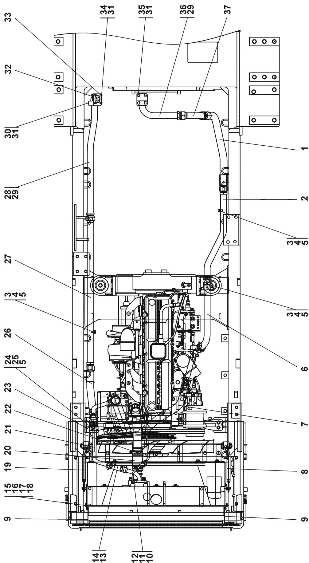
Рисунок 1.13 Система охлаждения Figure 1.13 Cooling system
