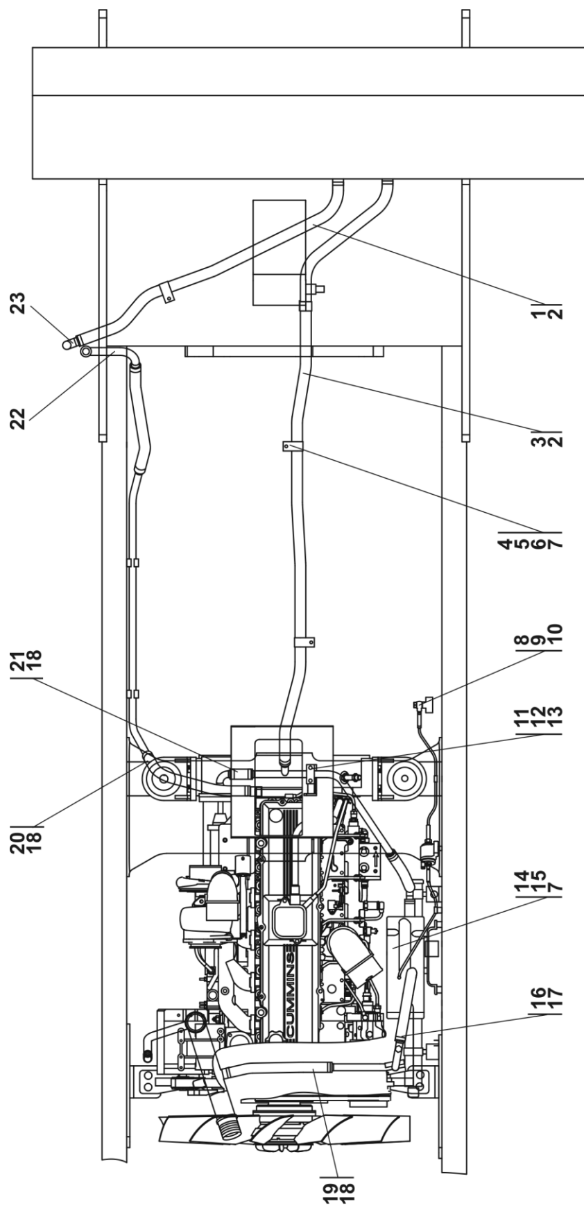
Рисунок 1.10 Установка системы подогрева Figure 1.10 Heating system mounting
