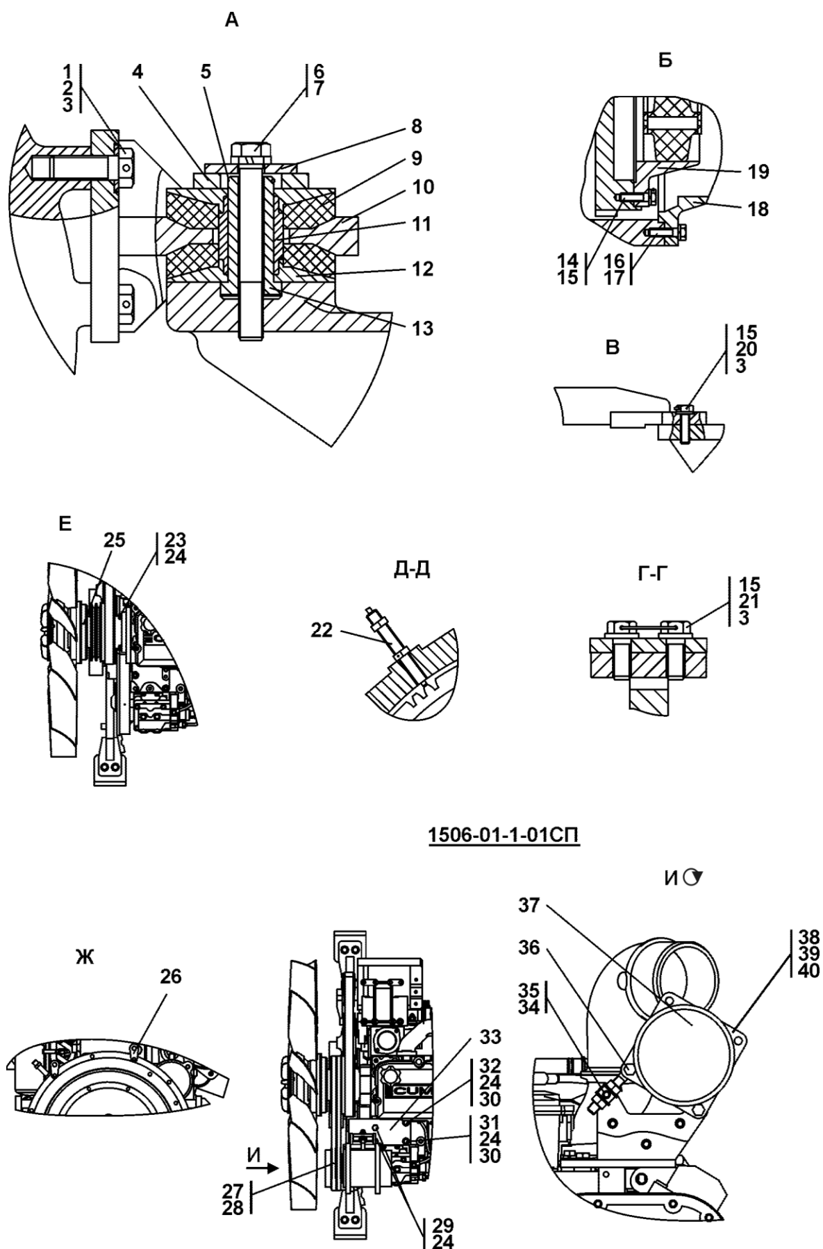
Рисунок 1.2 Установка двигателя QSC8,3-C245 «Cummins» Figure 1.2 QSC8,3-C245 «Cummins» engine mounting
