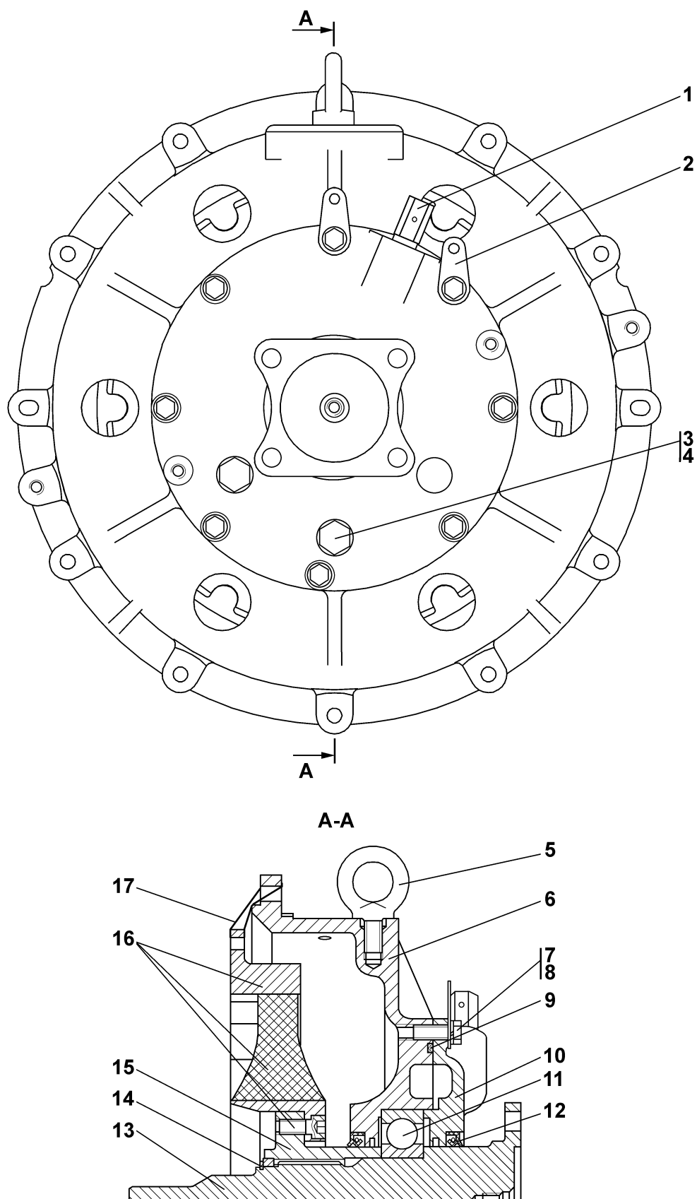
Рисунок 4.23 Муфта упругая Figure 4.23 Flexible coupling
