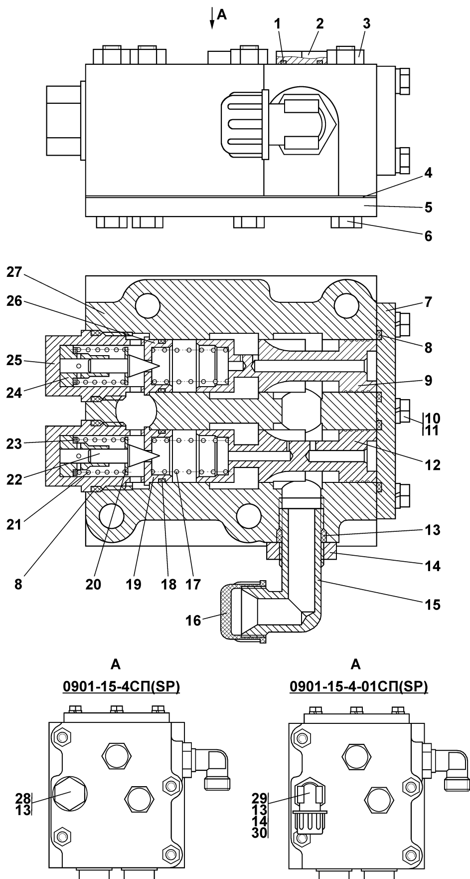
Рисунок 4.9 Клапан Figure 4.9 Valve
