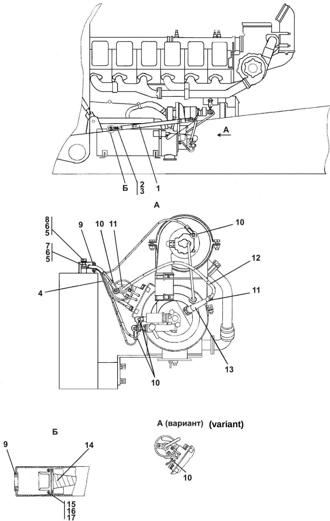
Рисунок 2.4 Электрооборудование подогревателя ПЖД600И Figure 2.6 PHZD600I heater electric equipment
