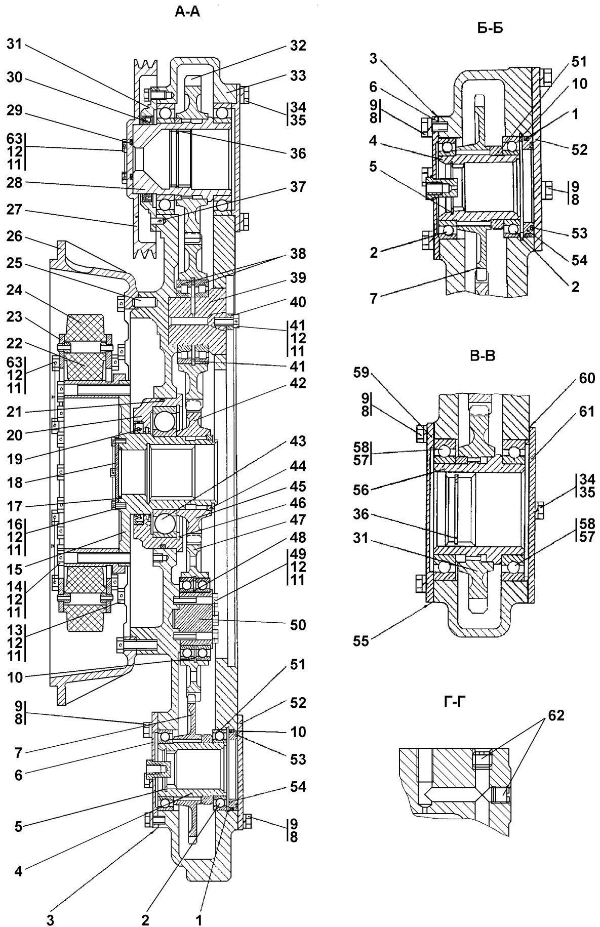
Рисунок 4.23 Редуктор привода насосов Figure 4.23 Pump drive reduction gear
