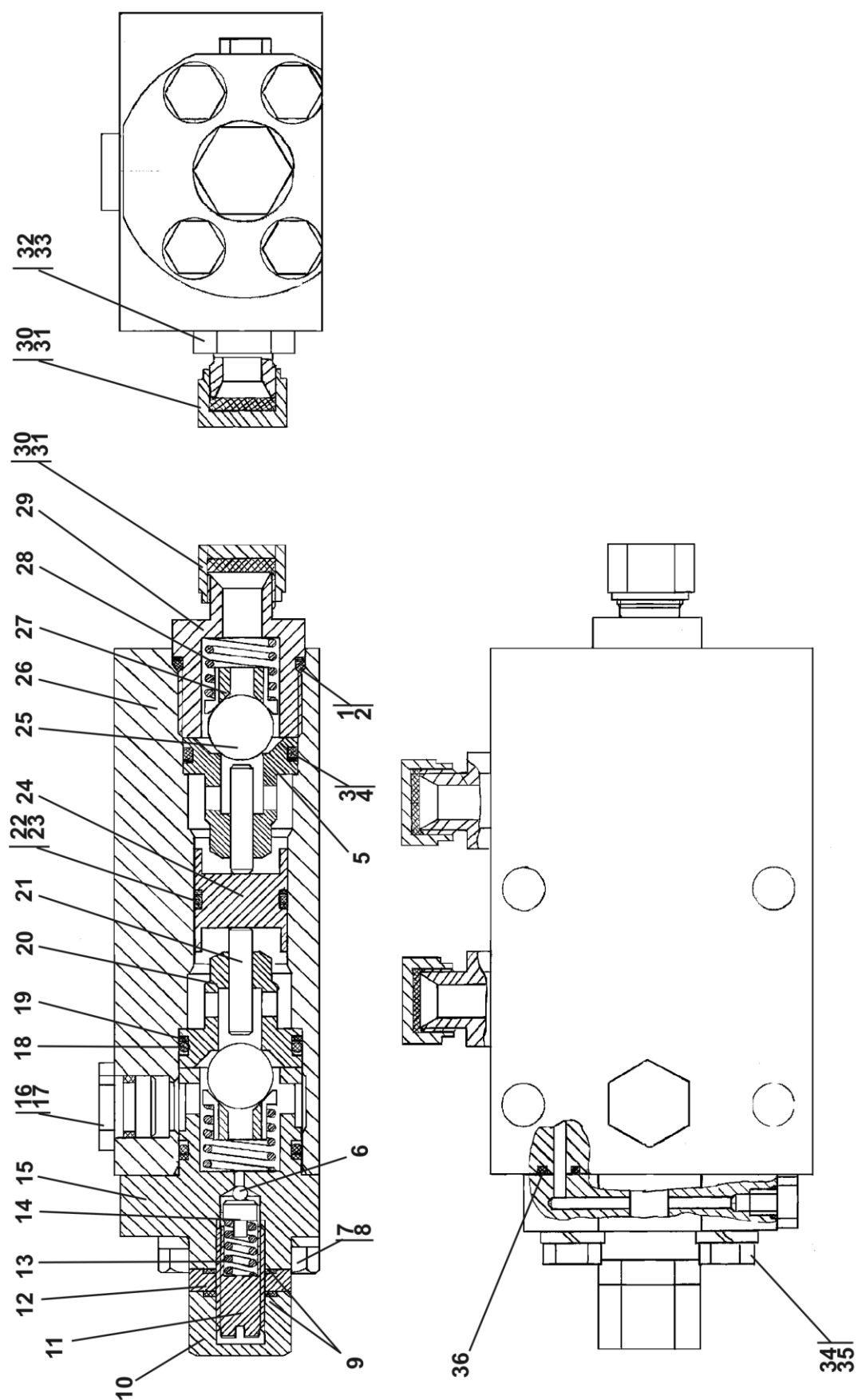
Рисунок 7.11 Гидрозамок Figure 7.11 Pilot controlled check valve
