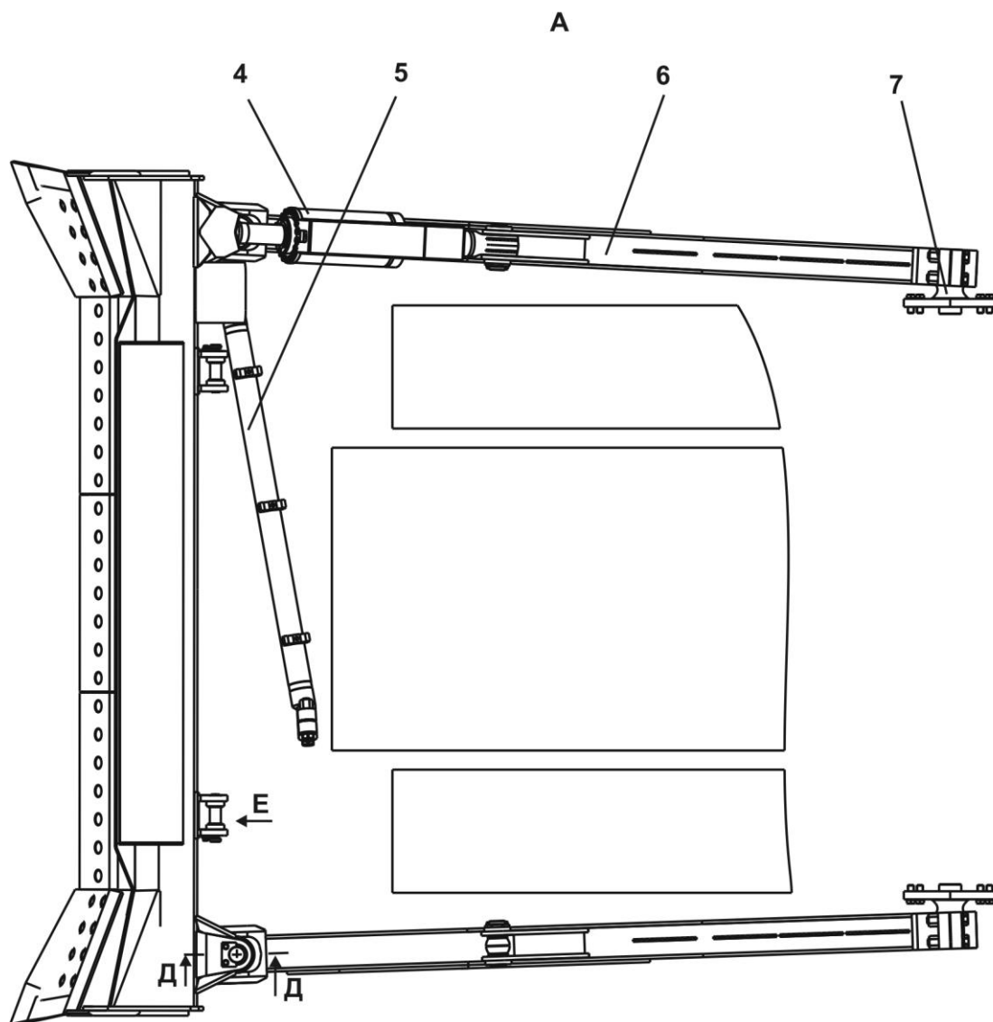
Рисунок 7.3 Оборудование бульдозерное Figure 7.3 Dozer equipment
