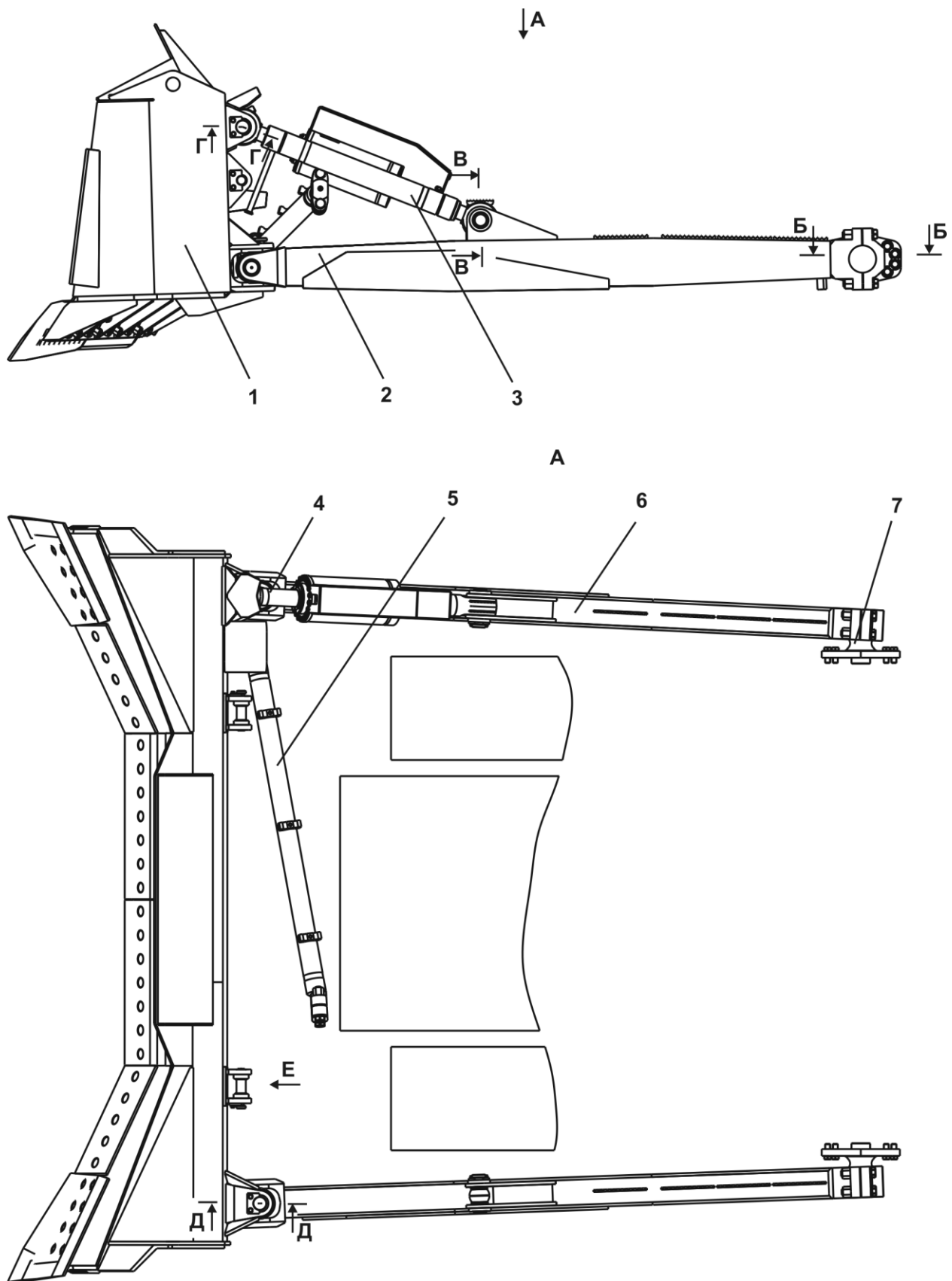
Рисунок 7.1 Оборудование бульдозерное сферическое
