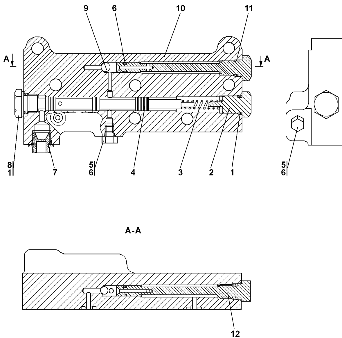
Рисунок 5.14 Клапан Figure 5.14 Valve
