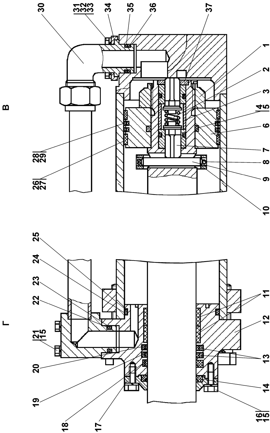
Рисунок 5.18 Гидроцилиндр Figure 5.18 Hydraulic cylinder
